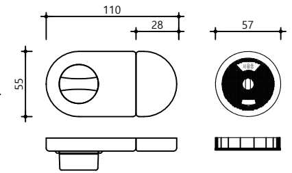
하드웨어 - 잠금쇠
