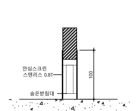
안심스크린 상세(전면부)
