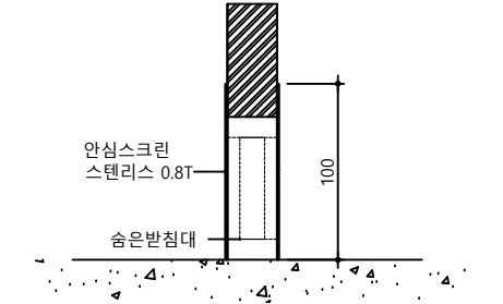
안심스크린(측면부)
