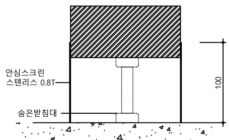
안심스크린 상세(전면부)
