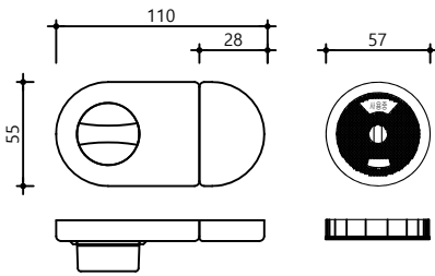
하드웨어 - 잠금쇠
