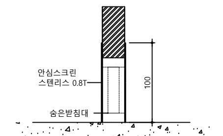
안심스크린(측면부)
