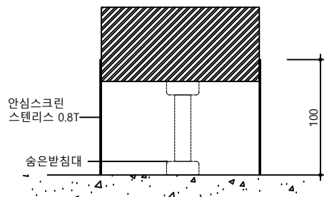
안심스크린 상세(전면부)
