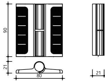
하드웨어 - 경첩
