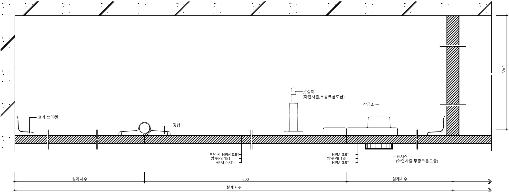
판넬 상세도
