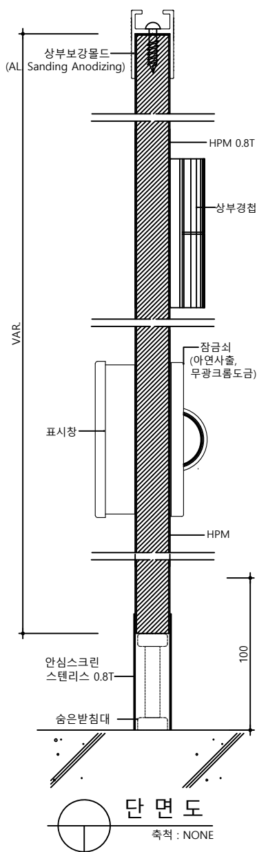
하드웨어 - 잠금쇠
