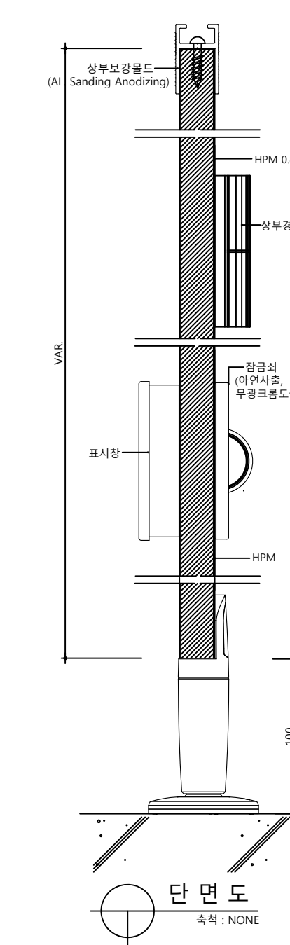
단면도
