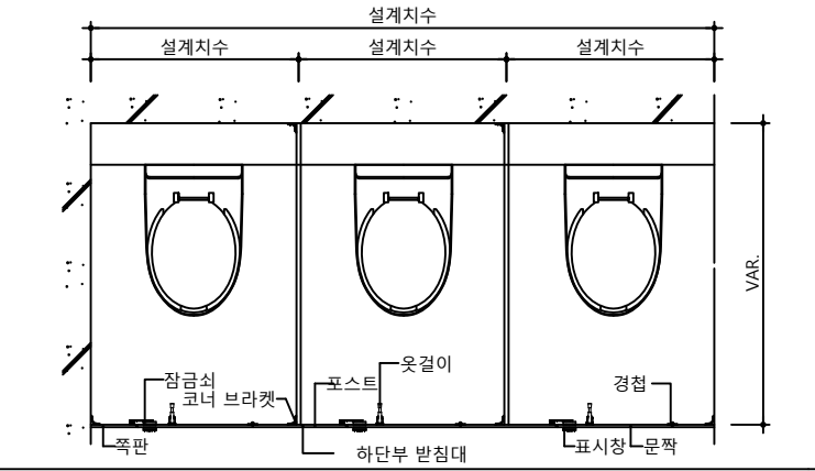
평면도
