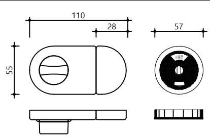
하드웨어 - 잠금쇠
