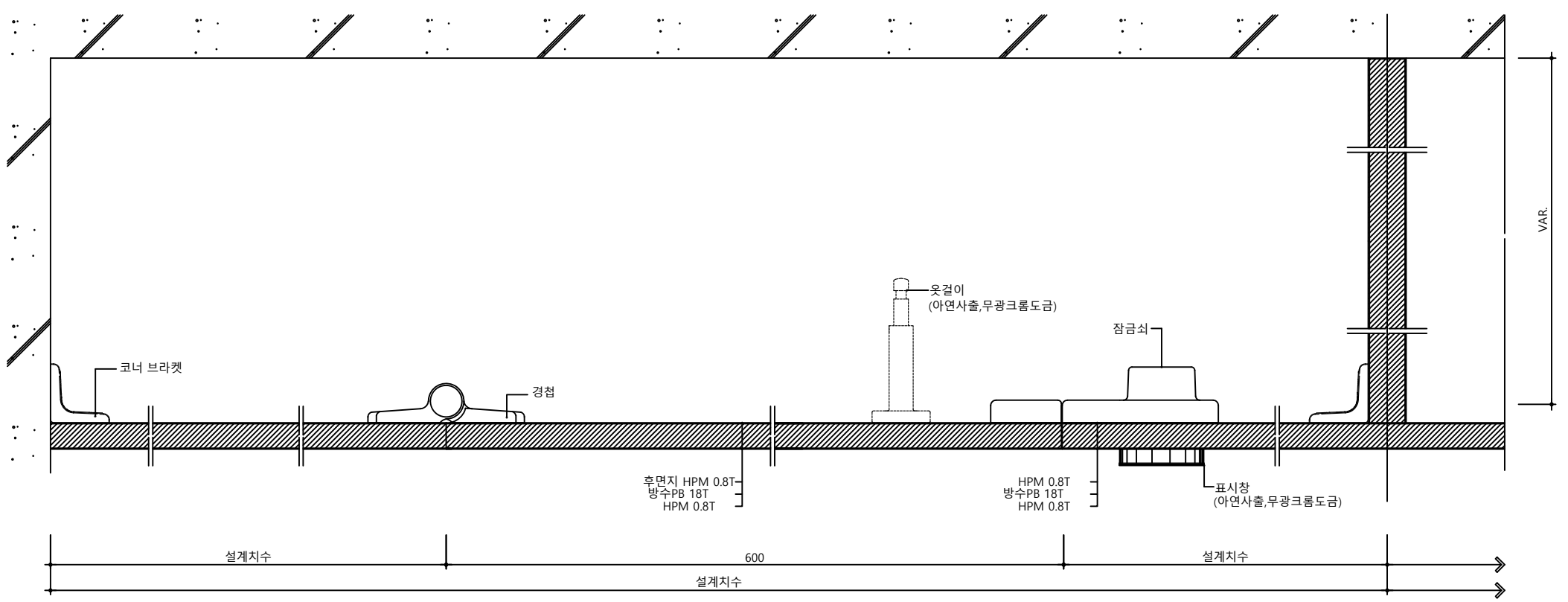
판넬 상세도
