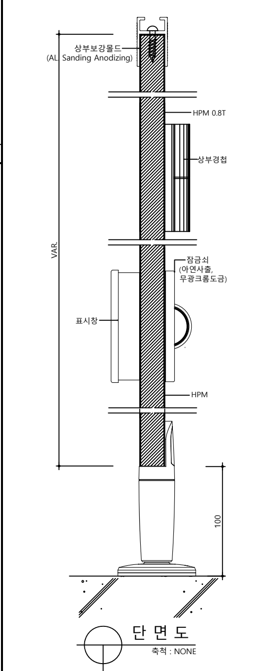
단면도
