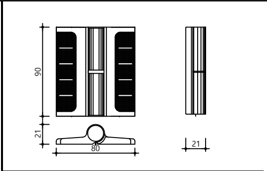
하드웨어 - 경첩
