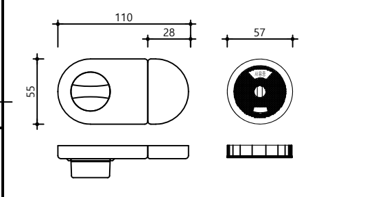
하드웨어 - 잠금쇠
