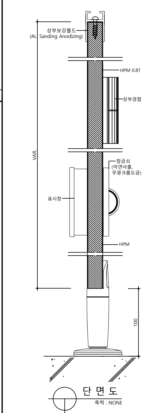
단면도
