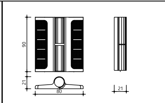
하드웨어 - 경첩
