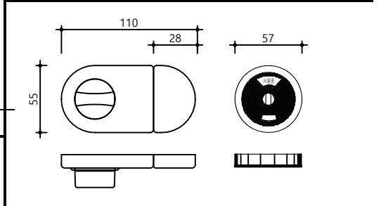
하드웨어 - 잠금쇠
