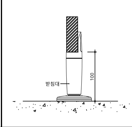
받침대 (측면부)
