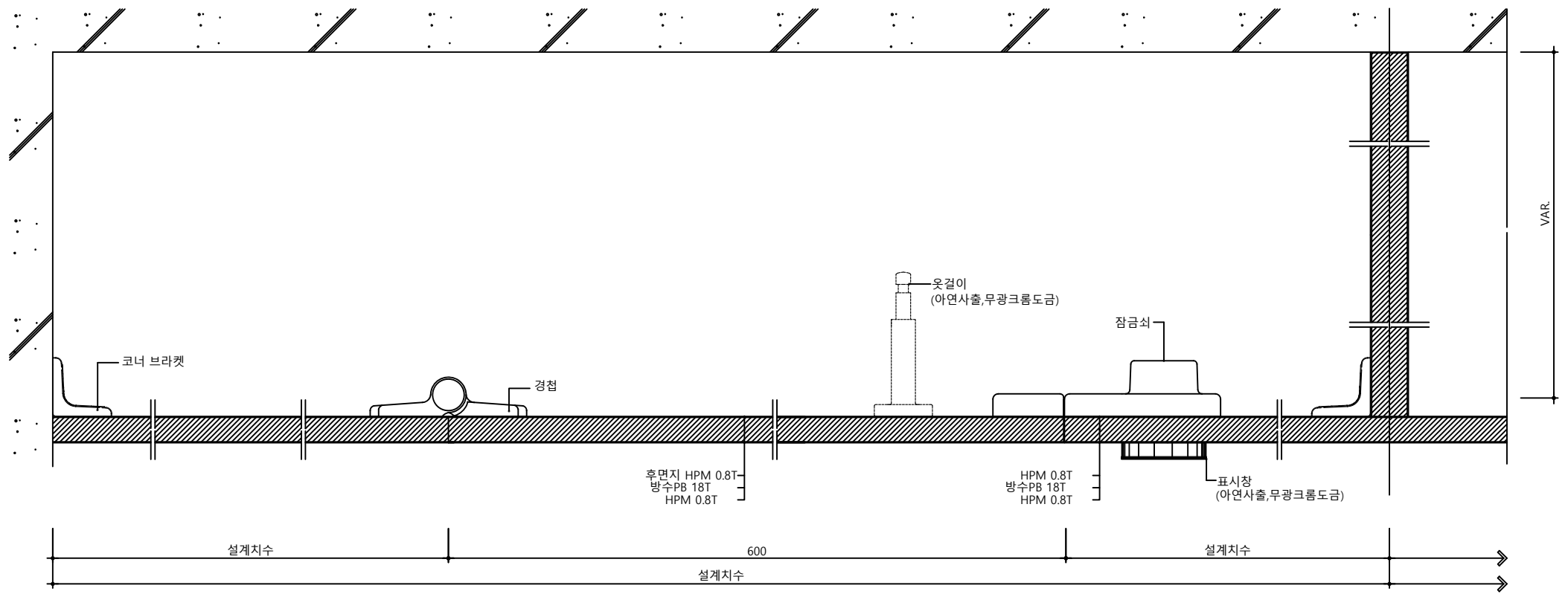
판넬 상세도
