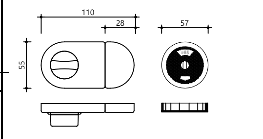
하드웨어 - 잠금쇠
