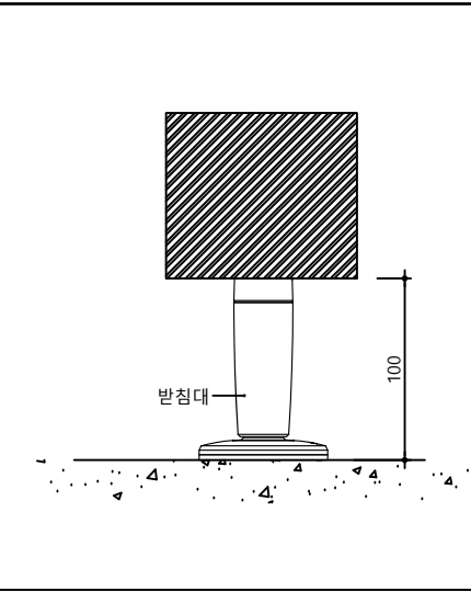
받침대 (전면부)
