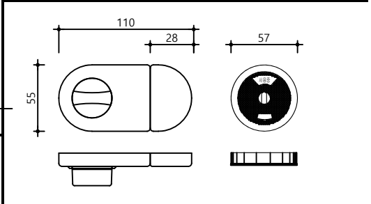
하드웨어 - 잠금쇠
