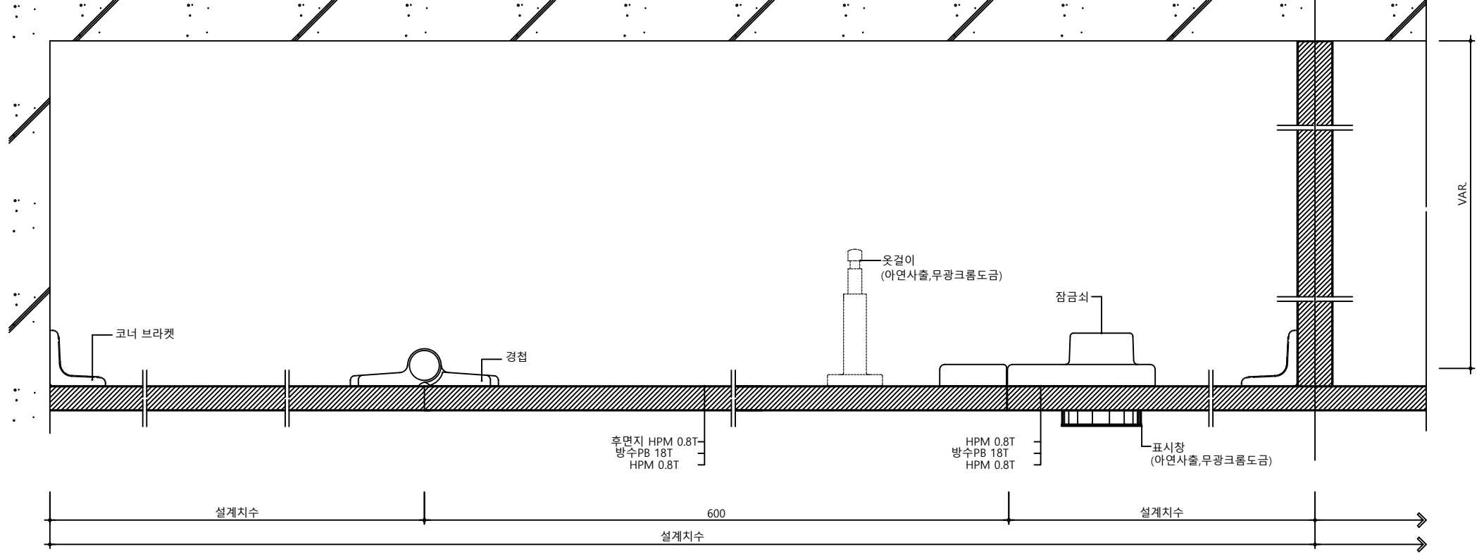
판넬 상세도
