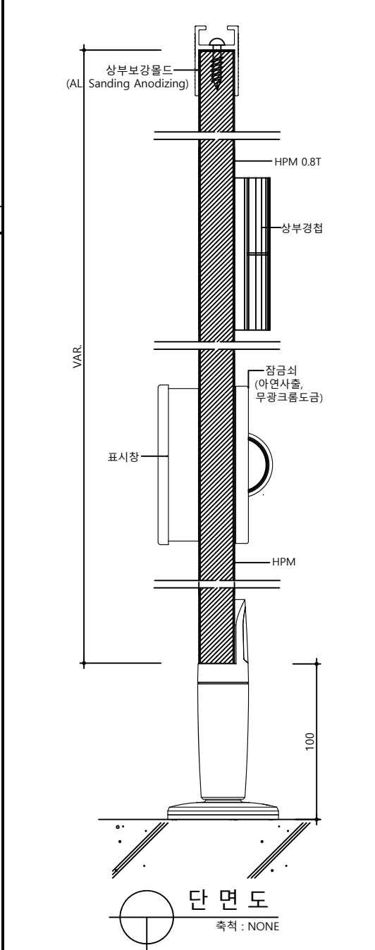
단면도
