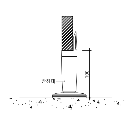
받침대 (측면부)
