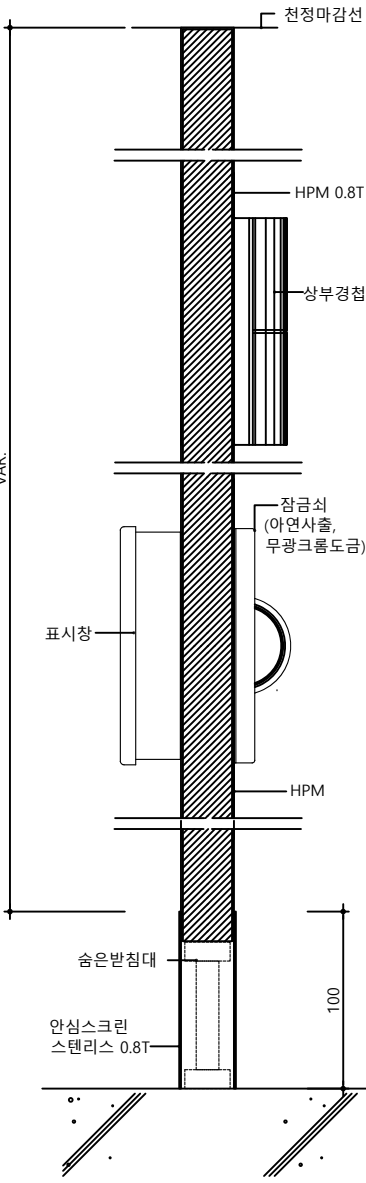
단면도 축척 : NONE
