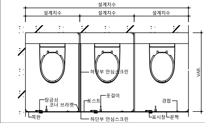
평면도
