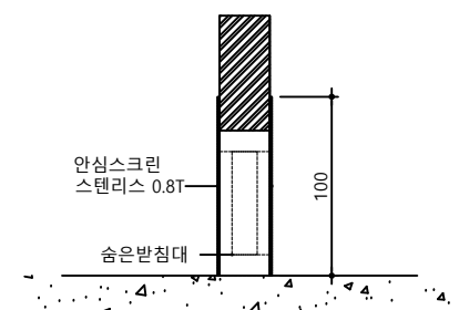
안심스크린 상세(전면부)
