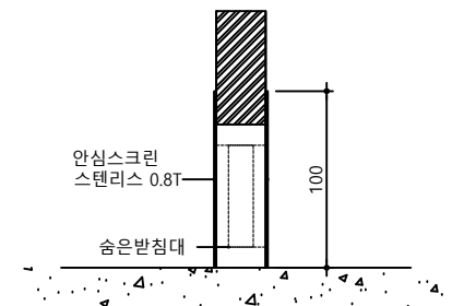
안심스크린(측면부)
