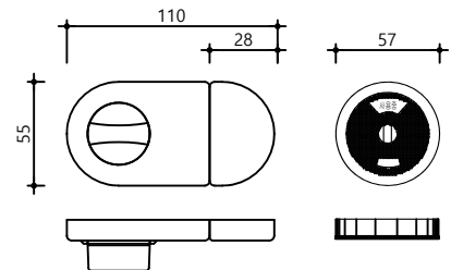
하드웨어 - 잠금쇠
