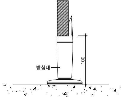
받침대 (측면부)
