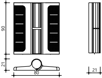
하드웨어 - 경첩
