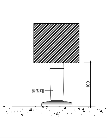
받침대 (전면부)
