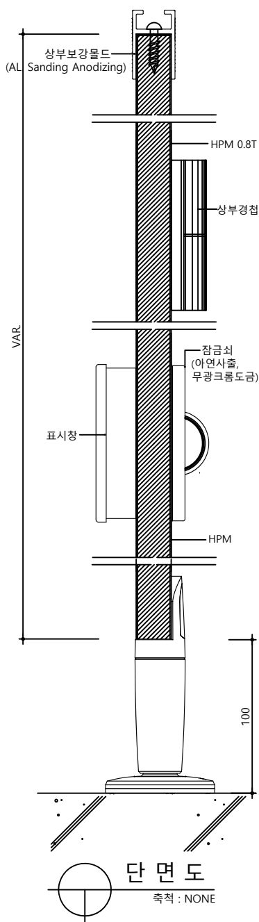
하드웨어 - 잠금쇠
