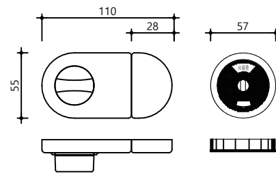
하드웨어 - 잠금쇠
