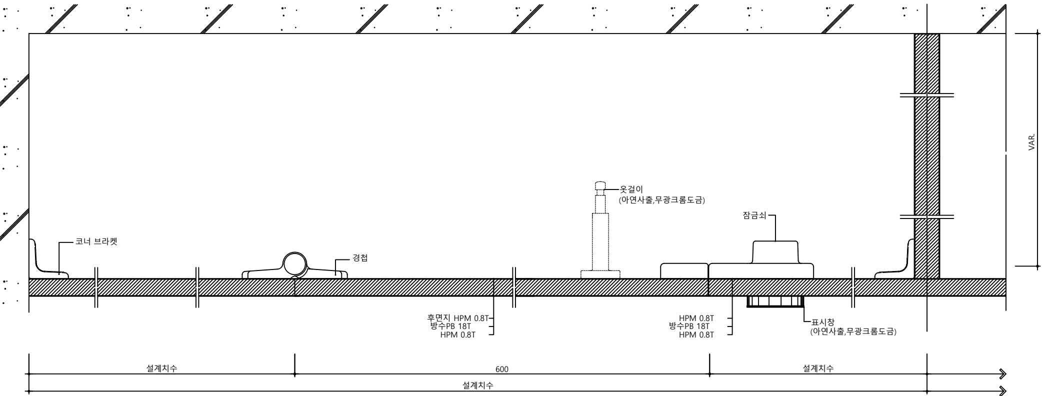
판넬 상세도
