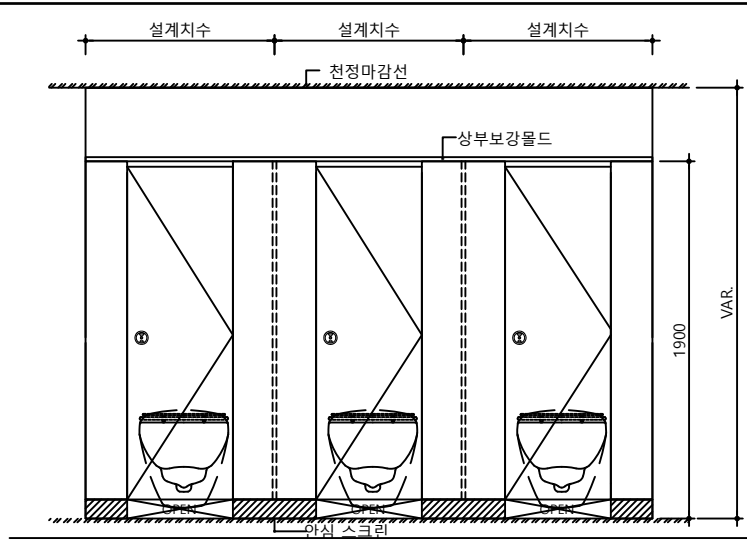
입면도 TYPE A
