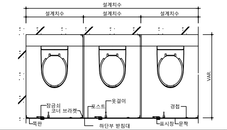
평면도
