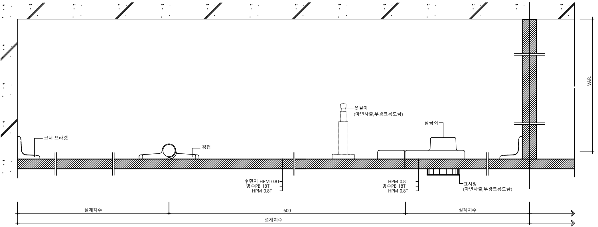
판넬 상세도
