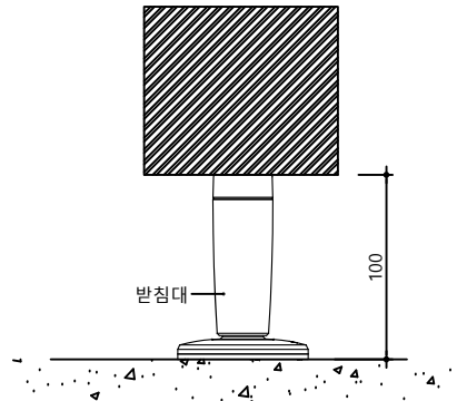
받침대 (전면부)
