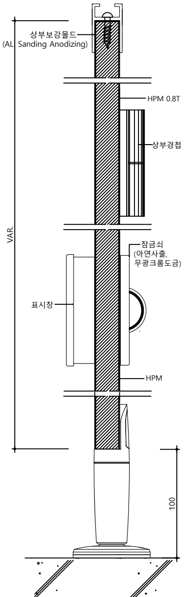
단면도
