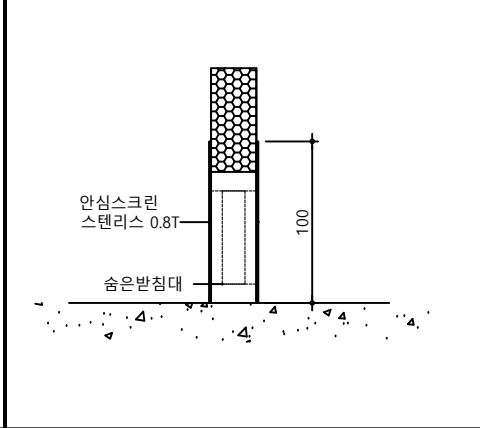
안심스크린(측면부)
