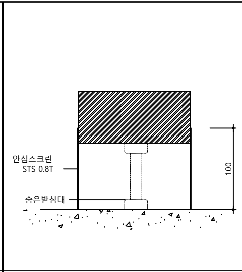
안심스크린 상세(전면부)
