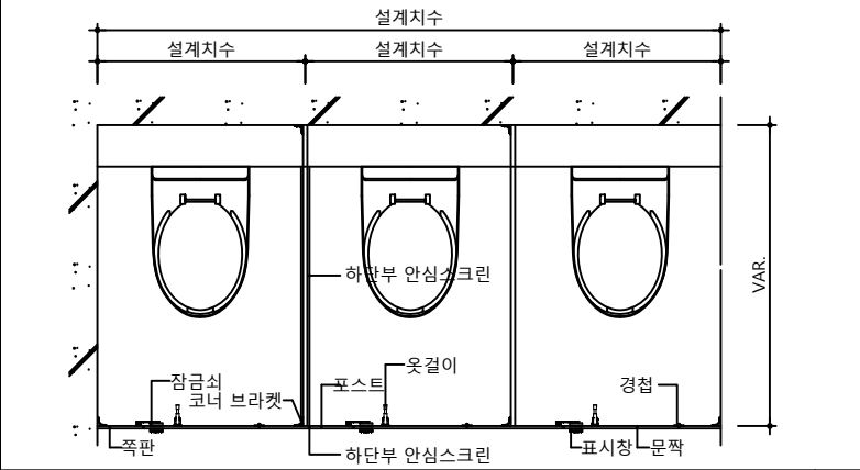
평면도
