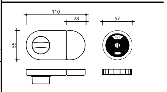
하드웨어 - 잠금쇠
