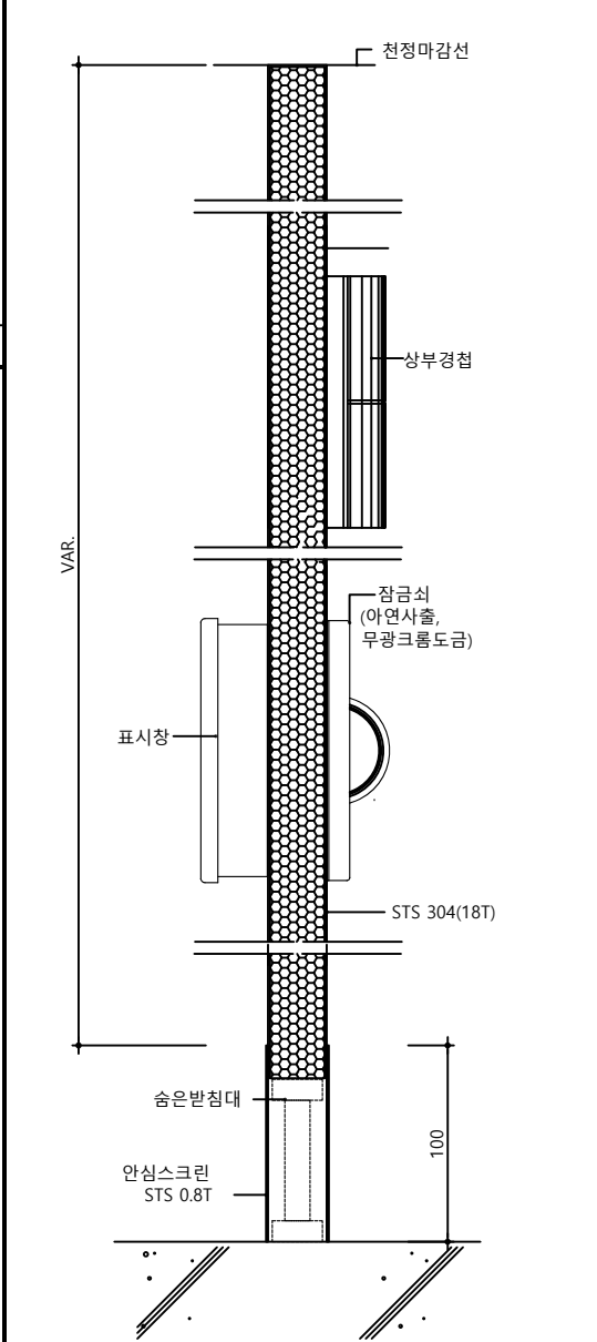
단면도
