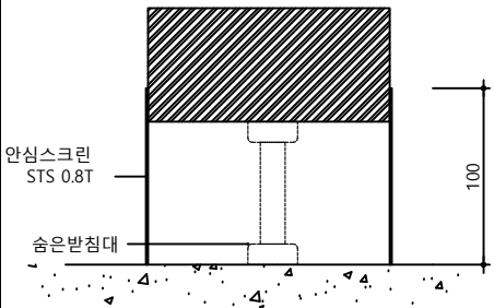
안심스크린 상세(전면부)
