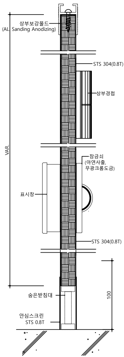
단면도 축척 : NONE
