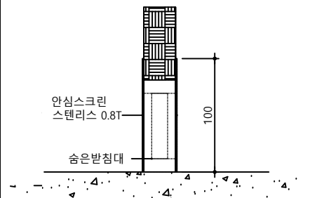
안심스크린(측면부)
