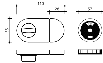
하드웨어 - 잠금쇠
