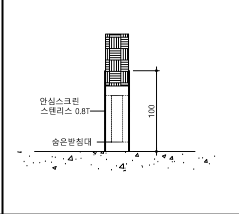
안심스크린(측면부)
