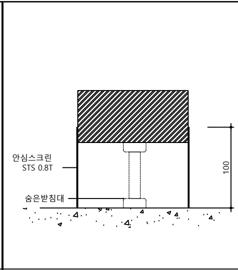
안심스크린 상세(전면부)
