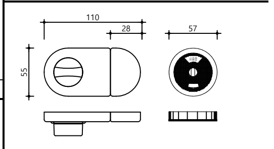
하드웨어 - 잠금쇠
