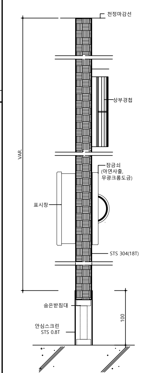
단면도
