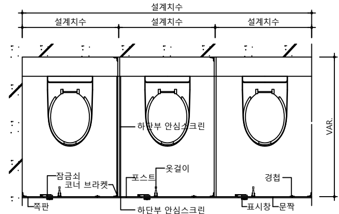
평면도
