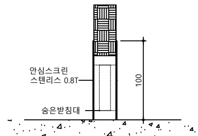
안심스크린(측면부)
