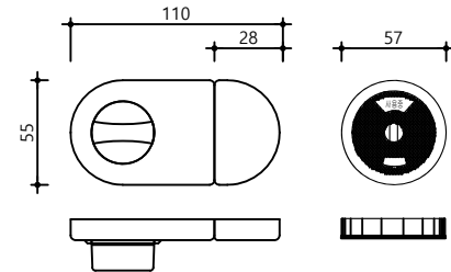
하드웨어 - 잠금쇠
