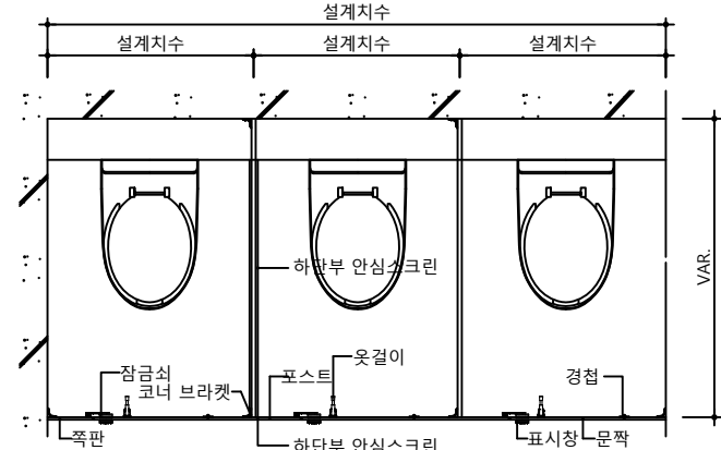
평면도
