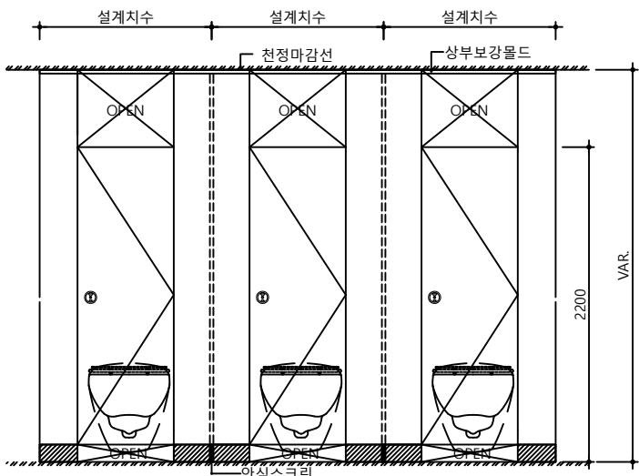
입면도 TYPE A
