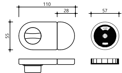
하드웨어 - 잠금쇠
