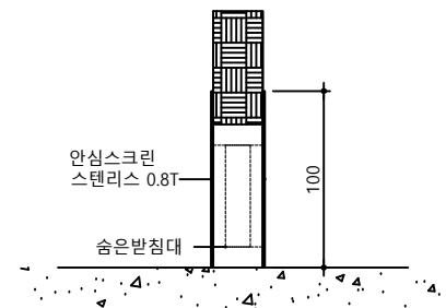
안심스크린(측면부)
