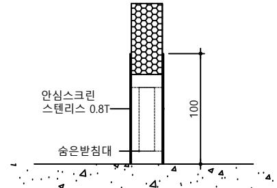
안심스크린(측면부)
