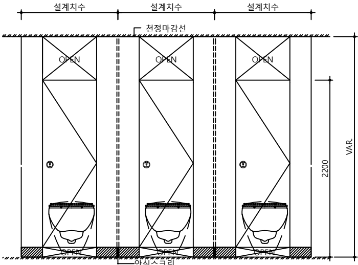
입면도 TYPE A
