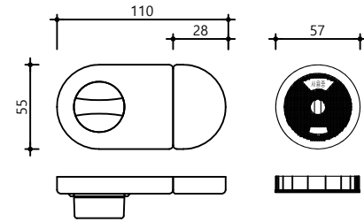
하드웨어 - 잠금쇠
