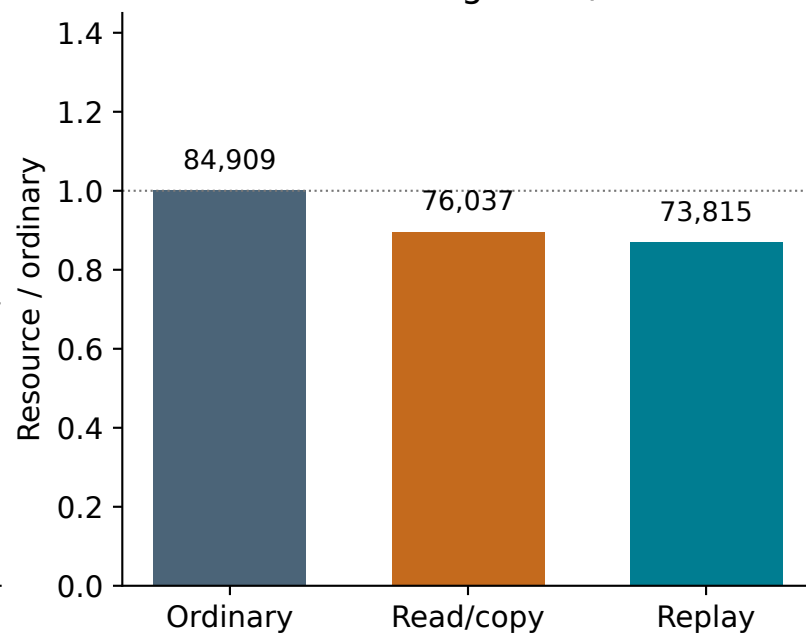
Vivado · Registers / FFs
