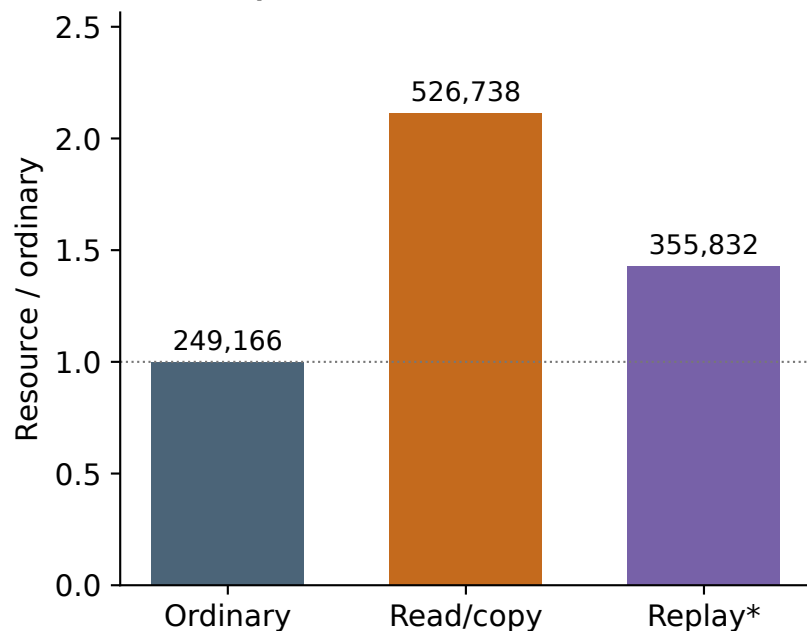
Vivado · CLB LUTs
