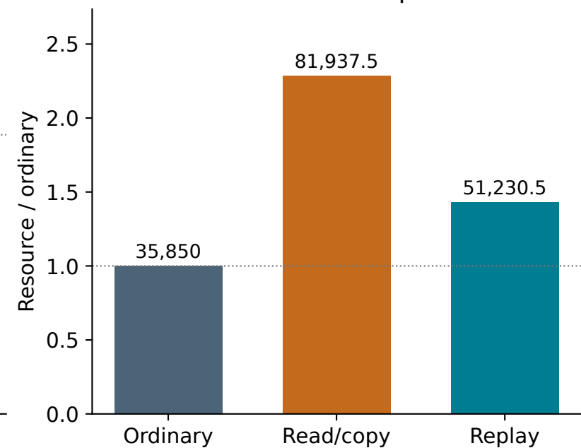
Vivado · BRAM36 equivalents
