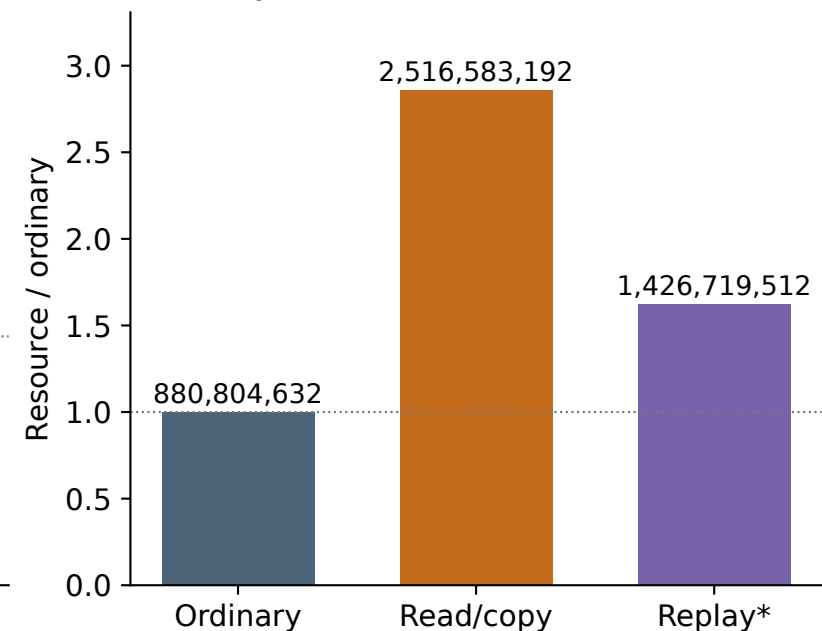
Vivado · BRAM36 equivalents
