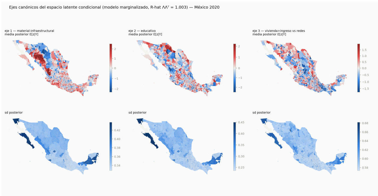
Figura 5. Los tres ejes canónicos del espacio latente condicional: media posterior E[z|Y] (arriba) y desviación posterior (abajo) por municipio, modelo marginalizado convergido ( \hat{R} \Lambda\Lambda^T = 1.003 ).
