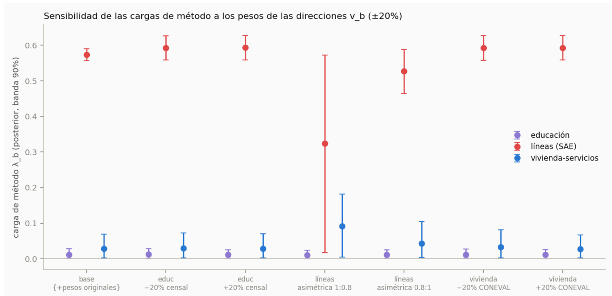
Figura E1. Sensibilidad de las cargas de método a los pesos de las direcciones v_b : la carga del bloque de líneas (rojo) es estable salvo cuando se desvía su propia dirección hacia la línea general ( \{1, 0.8\} ), donde la posterior se desestabiliza.
