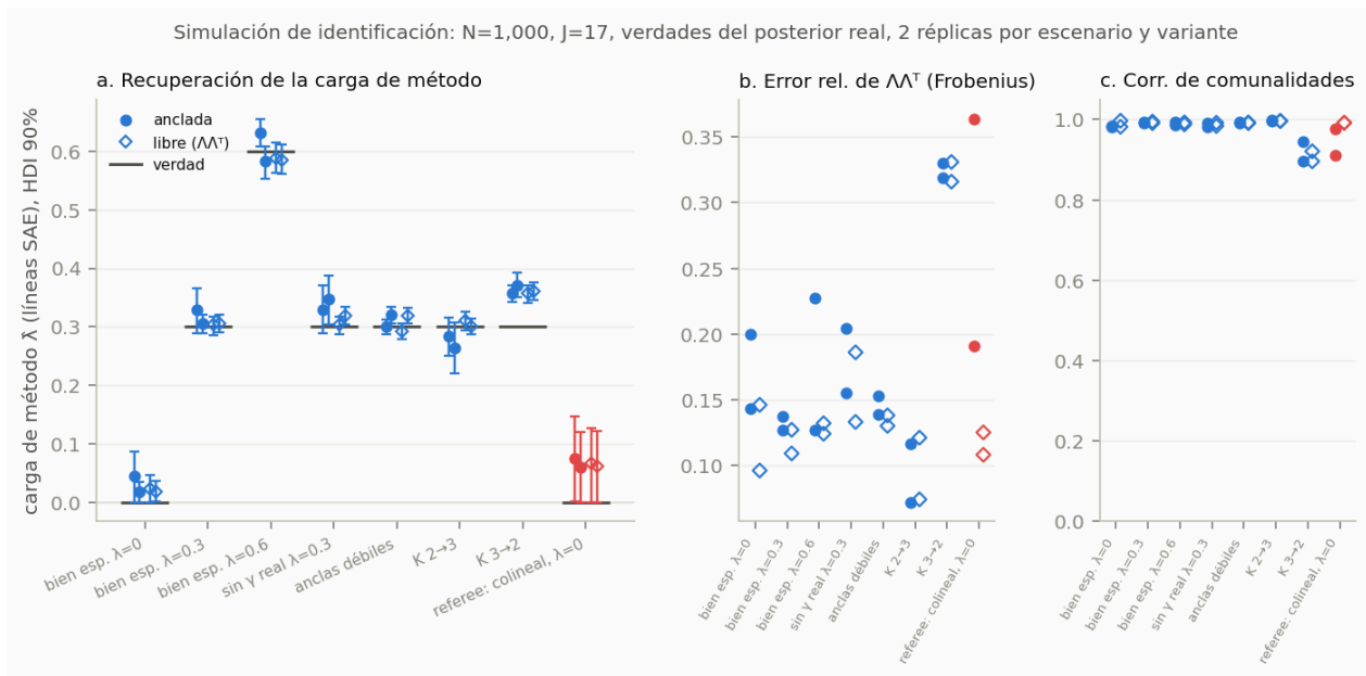
Figura F1. Simulación de identificación (N=1,000, J=17, verdades del posterior real). (a) Recuperación de la carga de método por escenario, parametrización anclada y libre, con la verdad marcada; el escenario del referee (colinealidad 0.98, \lambda=0 ) no fabrica la carga. (b) Error de Frobenius relativo de \Lambda\Lambda^T . (c) Correlación de comunalidades. La sub-extracción (K 3→2) es el único escenario que sesga materialmente.
