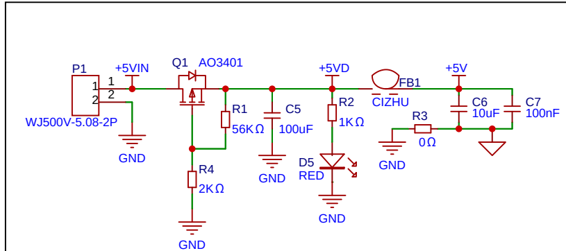
防反接电路
