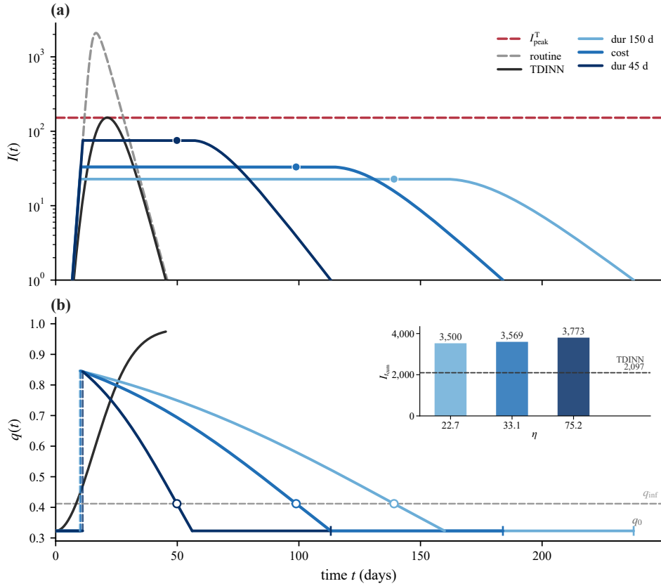
图 21: \eta 杠杆: 固定有效人口 N_{\text{eff}} = 2 \times 10^4 , 沿三条由引理 8.1 的理论口径得到的边界参照线取阈值 \eta = \theta N_{\text{eff}} 的情景一阈值控制轨迹。各条平台的高度即其 \eta ; 按 \eta 升序, 三条参照线依次为 dur 150 d ( \theta_{\text{dur150}} = 1.137 \times 10^{-3} , \eta = 22.7 )、cost ( \theta_{\text{cost}} = 1.656 \times 10^{-3} , \eta = 33.1 )、dur 45 d ( \theta_{\text{dur45}} = 3.762 \times 10^{-3} , \eta = 75.2 )。 (a) 社区感染者 I(t) (对数纵轴): 三条平台分别贴合各自的 \eta , 且因 N_{\text{eff}} < N^*(45\text{d}) 全部落在 I_{\text{peak}}^T 之下 (红虚线)。平台上的同色实心圆为 q_c(t) 拐点时刻 t_{\text{inf}} 在 I(t) 上的投影 ( t_{\text{inf}}, \eta ), 并非 I(t) 自身的拐点。在本文的单一口径下启动时间 t_1 随 N_{\text{eff}} 变 (本图 N_{\text{eff}} = 2 \times 10^4 处三条参照线依次为 9.92/10.29/11.12 d), 故绝对 t_{\text{inf}} 在不同 N_{\text{eff}} 图之间平移; 平台内相对位置 \lambda = (t_{\text{inf}} - t_1)/(t_2 - t_1) \approx 0.861 以及距平台结束的时间 t_2 - t_{\text{inf}} \approx 20.8/14.3/6.3 d (依次对应 dur 150 d/cost/dur 45 d) 基本不随 N_{\text{eff}} 改变 (见附录 A)。灰虚线为同一 N_{\text{eff}} 下的常规控制, 其峰值 \approx 0.105 N_{\text{eff}} 、到动态清零的总累计感染 \approx 0.348 N_{\text{eff}} ——两者都是与池规模无关的固定比例 (随 N_{\text{eff}} 线性放大, 此处 N_{\text{eff}} = 2 \times 10^4 即 2093/6970); 其中累计约为右上角 inset 中策略柱的两倍, 若入柱图会压扁三条策略柱的排序, 故只以闭式给出、不在图中另绘; 黑实线为 TDINN 在西安全市口径下的原始拟合轨迹 (峰值 151.90、清零 45.27 d), 作为固定拟合参照, 不随 N_{\text{eff}} 重算 (见第 8 节 TDINN 基准的口径说明)。 (b) 隔离率 q_c(t) : 三条松弛曲线与 TDINN 的上升高斯 q_{\text{TDINN}}(t) ; 各条彩色实线均包含控制前和 t_2 后直到自身动态清零的 q_0 = 0.3230 阶段, 以及 t_1 \leq t \leq t_2 的阈值控制段; 彩色垂直虚线连接 t_1 处从 q_0 到 q_c(t_1^+) 的瞬时跳跃。曲线按动态清零时刻从长到短叠绘, 使短清零轨迹在重合的 q_0 段上优先可见; 各曲线在 q_0 上的同色短竖线标出自身动态清零时刻; 灰虚线为拐点高度 q_{\text{inf}} = 1 - 1/[2(1 - \beta)] = 0.4119 。白心圆为各条曲线的凹凸拐点, 均落在 q_{\text{inf}} 上, 与其只依赖 \beta 、不依赖 ( N_{\text{eff}}, \eta ) 的结论一致。右上角内嵌柱图按 \eta 递增排列, 给出动态清零 I(t) \leq 1 时的总累计感染 I_{\text{cum}} , 柱色随 \eta 加深, 纵轴从零起算; 黑虚线为 TDINN 全市固定拟合参照 I_{\text{cum}}^T = 2096.76 。三条均高于该参照且随 \eta 递增; 此处 N_{\text{eff}} = 2 \times 10^4 已超过累计占优临界 N_{\text{cum}, \infty}^* \approx 1.17 \times 10^4 (推论 8.5 及第 8.5 节), 故累计约束在三条上均不成立。
