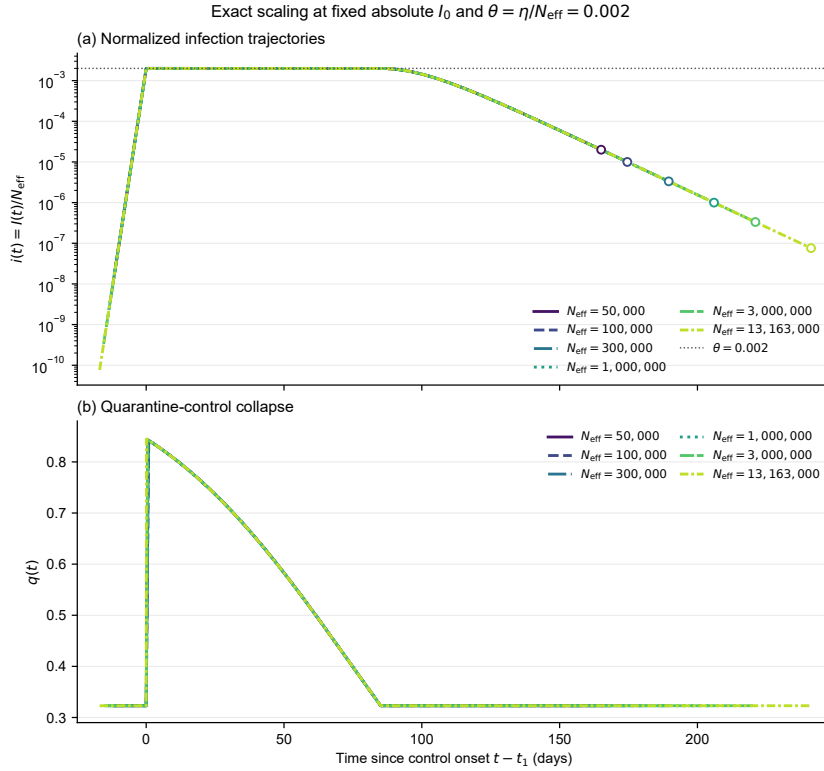
图 18: 固定绝对初值 I_0 与 \theta = 0.002 时不同 N_{\text{eff}} 的归一化感染轨迹 i 与隔离率 q 在平移时间 t - t_1 上的折叠 ( i_0 = I_0/N 随 N 变，故 t_1 由 11.39 升到 16.90 天；引理不含绝对时刻， t - t_1 是恰当基准)。白心圆为各 N_{\text{eff}} 下绝对判据 I = 1 对应的不同清零终点。
