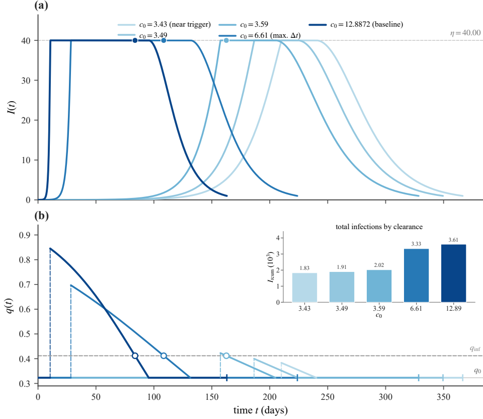
图 23: 固定 N_{\text{eff}} = 2 \times 10^4 、 \theta = 0.002 ( \eta = 40 )、西安传播参数，沿 c_0 取五个代表值的阈值控制轨迹。(a) I(t) : 平台同高为 \eta ， c_0 增大使 t_1 提前、上升支变陡；实心圆为 q_c(t) 拐点时刻 t_{\text{inf}} 在平台上的投影 ( t_{\text{inf}}, \eta )，非 I(t) 自身拐点。(b) q_c(t) : q_{\max} 随 c_0 展开，白圈（内部拐点）全部落在 q_{\text{inf}} = 0.4119 ； c_0 = 3.43, 3.49 因 q_{\max} < q_{\text{inf}} 全程凸、无内部拐点。右上柱图为各情景到自身动态清零 I(t) = 1 的总累计感染 I_{c,\text{cum}} = I_{c,\text{cum}} + I_{q,\text{cum}} ，在这五个代表点上随 c_0 递增。不画 TDINN 与常规控制： c_0 改变了接触结构，固定参照不可比。
