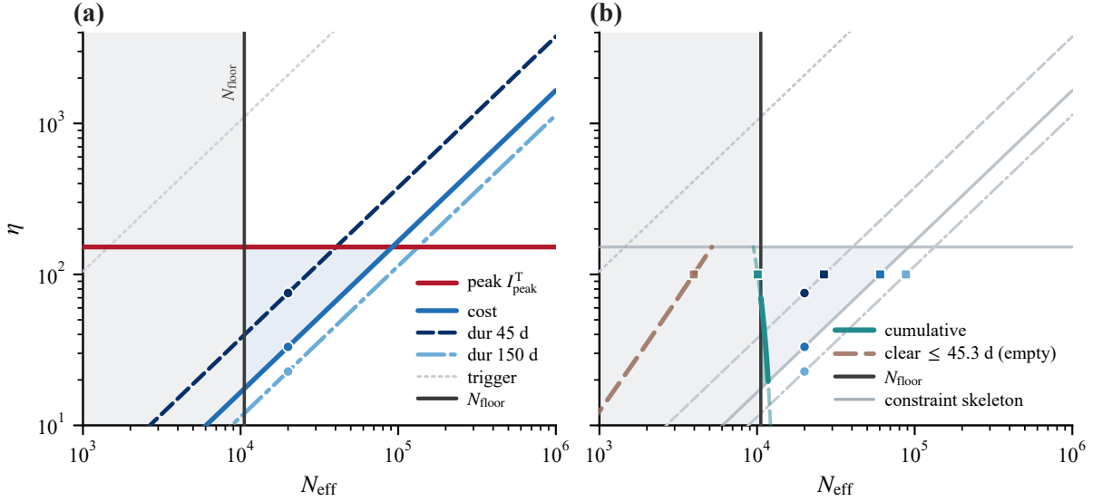
图 20: (N_{\text{eff}}, \eta) 平面上情景一阈值控制相对 TDINN 全市固定拟合参照的占优区域，双对数坐标。(a) 直线族（强度量）：峰值线 \eta = I_{\text{peak}}^T = 151.90 （红）、成本线 \eta = \theta_{\text{cost}} N （蓝）、两条时长线 \eta = \theta_{\text{dur}}(T_{\max}) N （45 d 虚线、150 d 点划线）与触发线 \eta = i_{\text{max}}^{\text{no}} N （点线， i_{\text{max}}^{\text{no}} = 0.1047 ）。阴影为占优楔形 \mathcal{W}_{\text{pcd}} ，以成本线为下界，对应 T_{\max} \rightarrow \infty 口径，顶点 N_{\infty}^* \approx 9.17 \times 10^4 ；由 \theta_{\text{dur}}(T) T \approx 0.170 ， T_{\max} \lesssim 103 d 时改由时长线绑定，例如 N^*(45\text{d}) \approx 4.04 \times 10^4 。(b) 弧线族（广延量）：累计边界（蓝青， Nh = I_{\text{cum}}^T ）在图示范围内自 (9471, 151.90) 延伸至 (12177, 10)，其中 \eta = 10 是绘图区间下限而非等值线的自然终点；清零边界（暖灰棕， t_{\text{end}} = t_{\text{end}}^T ，自 (865.9, 10) 到 (5165.7, 151.90)）。累计弧在 (11762, 19.48) 穿出楔形，其后一段以淡虚线示意等值线延续但不再构成 \mathcal{W}_{\text{cum}} 的边界。两面板中的竖直实线为最小相容易感池 N_{\text{floor}} = 1.06 \times 10^4 （式 (8.10)），其左侧斜纹区与观测不相容；清零弧全段位于该线左侧（最大值 N = 5166 ），故清零占优区为空集、全线以虚线绘出；累计占优区收缩为 N \in [1.06, 1.18] \times 10^4 的窄条。骨架线（峰值·成本·时长·触发）以中性灰重绘以突出弧线。两面板的圆点与方点分别对应图 21 与图 22 的采样角色，同色联动。 \eta = 100 处 N_{\text{cum}} \approx 1.010 \times 10^4 、 N_{\text{clr}} \approx 3.97 \times 10^3 。
