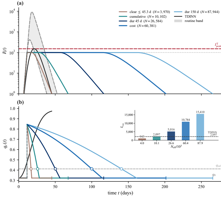
图 22: N 杠杆: 固定绝对阈值 \eta = 100 , 在五个有效人口下的情景—阈值控制轨迹。五条平台高度相同 (均为 \eta ), 故 N_{eff} 无法在纵轴上直读, 各曲线对应的 N_{eff} 已随角色名列于图例; 五个取值取自各条边界与 \eta = 100 的交点: clear \leq 45.3 d ( N_{eff} = 3,970 )、cumulative (10,102)、dur 45 d (26,584)、cost (60,381)、dur 150 d (87,944)。其中 clear 成员的平台仅 \Delta t = 6.3 d, 近于退化。(a) I(t) (对数纵轴): 五条平台全部恒在 \eta = 100 (灰虚线), 与池规模无关, 这是强度量只通过 \theta = \eta/N_{eff} 进入的直接体现; 平台时长则随 N_{eff} 增大而显著拉长。灰色带为常规控制在 N_{eff} \in [3,970, 87,944] (与上列五个取值同范围) 上取 8 条几何间隔轨迹的逐点最小-最大包络, 仅绘制到全部成员均未清零为止; 两条灰虚线为区间端点的代表轨迹。带宽即该反事实策略对池规模的敏感度, 与阈值控制平台的零带宽形成对照。带内每条常规控制的峰值 \approx 0.105 N_{eff} 、到动态清零的总累计感染 \approx 0.348 N_{eff} , 均为与池规模无关的固定比例 (随 N_{eff} 线性放大, 最大成员 N_{eff} = 87,944 处约为 9200/30600); 其中累计约为 inset 中同规模策略柱的两倍, 故只以闭式给出、不在图中另绘。黑实线为 TDINN 在西安市口径下的原始拟合轨迹 (峰值 151.90、清零 45.27 d), 作为全市固定拟合参照只画一条, 不随 N_{eff} 重算; 红虚线为其峰值 I_{peak}^T 。(b) q_c(t) : 五条松弛曲线与 TDINN 的 q_{TDINN}(t) ; 每条彩色实线均包含控制前和 t_2 后直到自身动态清零的 q_0 阶段, 以及 t_1 \leq t \leq t_2 的阈值控制段, 彩色竖直虚线连接 t_1 处从 q_0 到 q_c(t_1^+) 的瞬时跳跃。曲线按动态清零时刻从长到短叠绘, 使短清零轨迹在重合的 q_0 段上优先可见; 各曲线在 q_0 上的同色短竖线标出自身动态清零时刻。白心圆的拐点同样全部落在 q_{inf} = 0.4119 , 给出跨 N_{eff} 的不变性, 与图 21 的跨 \eta 不变性互补。右上角内嵌柱图按 N_{eff} 递增排列, 给出动态清零 I(t) \leq 1 时的总累计感染 I_{cum} ; 五柱依次约为 945/2097/5016/10784/15410, 黑虚线为 TDINN 全市固定拟合参照 I_{cum}^T = 2096.76 。因此 clear 边界远低于该参照, cumulative 边界按定义恰好达到该参照, 而其余三条边界均高于该参照。
