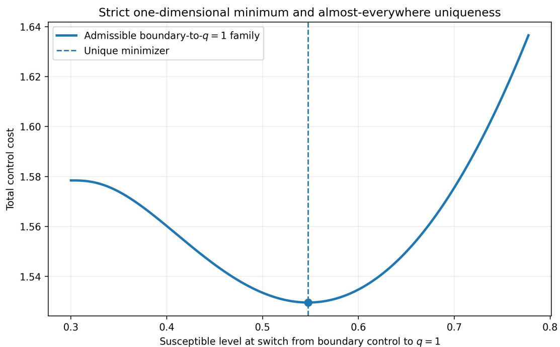
图 4: 容量转完全跟踪位置与总成本的关系。曲线展示一维策略族的严格极小; 解析依据为 (90) 及推论12.3, 图形本身不承担全局最优性证明。
