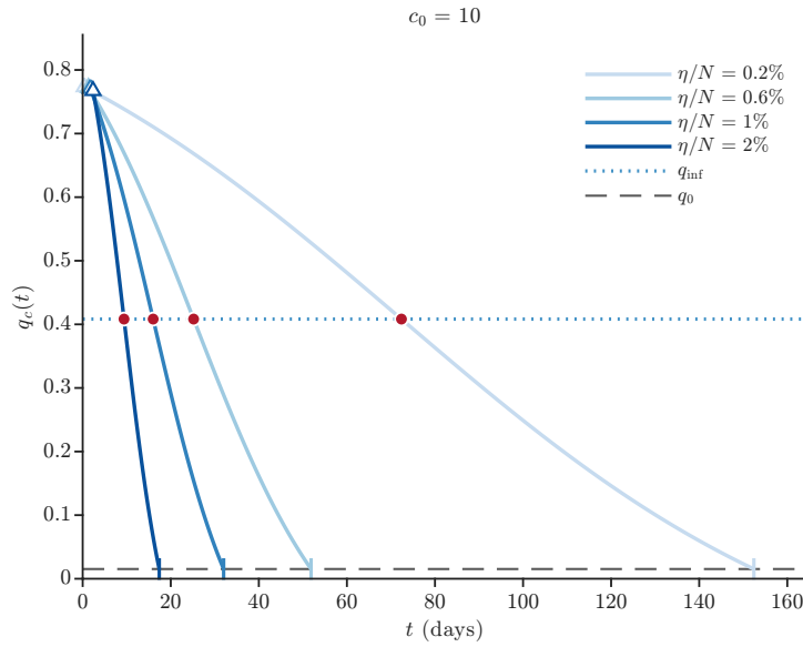
图 7: 固定 c_0 = 10 时, \eta/N = 0.2\%, 0.6\%, 1\%, 2\% 下隔离率 q_c(t) 的绝对时间轨迹。空心三角形和同色短竖线分别标出 t_1 和 t_2 ; 灰色虚线为 q_0 , 蓝色点线为 q_{\text{inf}} , 暗红圆点为内部拐点。
