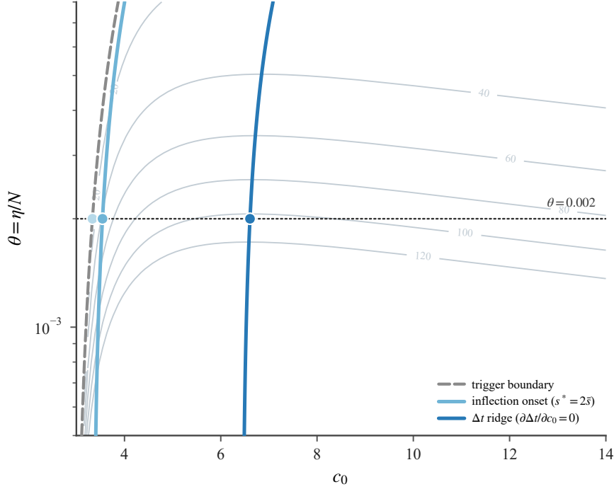
图 24: (\theta, c_0) 平面上阈值控制律的结构相图。三条曲线为触发边界 c_{0,\text{trig}}(\theta) 、内部拐点边界 s^* = 2\bar{s} 与控制时长脊线 \partial\Delta t/\partial c_0 = 0 ，灰色等值线为 \Delta t (天)。图 23 的三个代表 c_0 为三条边界与 \theta = 0.002 (点线) 的交点，同色圆点标出。本图仅报告结构量，不含占优边界，亦不画 J 或 \eta = I_{\text{peak}}^T 参照线。
