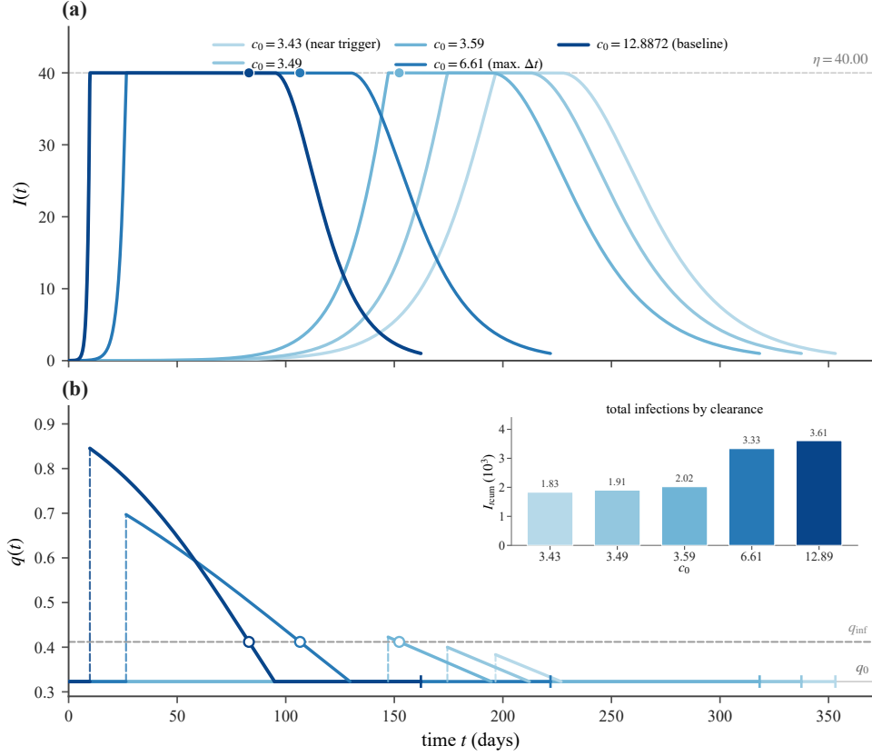
图 23: 固定 N_{\text{eff}} = 2 \times 10^4 、 \theta = 0.002 ( \eta = 40 )、西安传播参数，沿 c_0 取五个代表值的阈值控制轨迹。(a) I(t) : 平台同高 = \eta ， c_0 增大促使 t_1 提前、上升支变陡；实心圆为 q_c(t) 拐点时刻 t_{\text{inf}} 在平台上的投影 ( t_{\text{inf}}, \eta )，非 I(t) 自身拐点。(b) q_c(t) : q_{\max} 随 c_0 展开，白圈（内部拐点）全部落在 q_{\text{inf}} = 0.4119 ； c_0 = 3.43, 3.49 因 q_{\max} < q_{\text{inf}} 全程凸、无内部拐点。右上柱图为各情景到自身动态清零 I(t) = 1 的总累计感染 I_{\text{cum}} = I_{c, \text{cum}} + I_{q, \text{cum}} ，在这五个代表点上随 c_0 递增。不画 TDINN 与常规控制： c_0 改变了接触结构，固定参照不可比。
