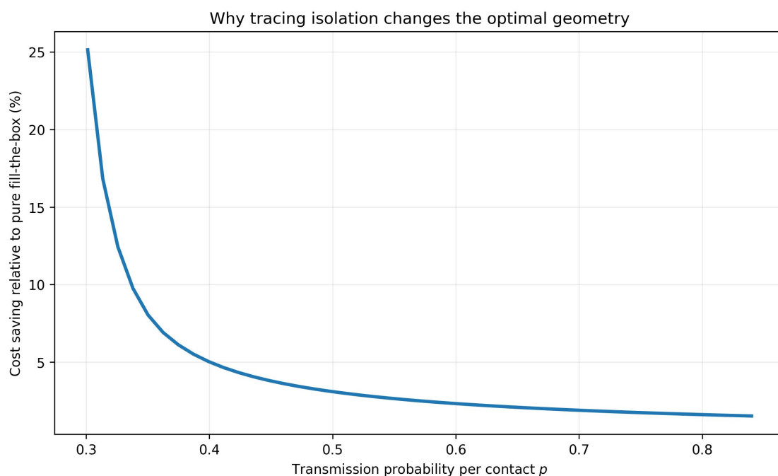
图 7: 原工程参数扫描中, 相对于纯容量填充的成本节省随传播概率变化的数值结果。该图不构成对所有参数的严格比较静态结论。
