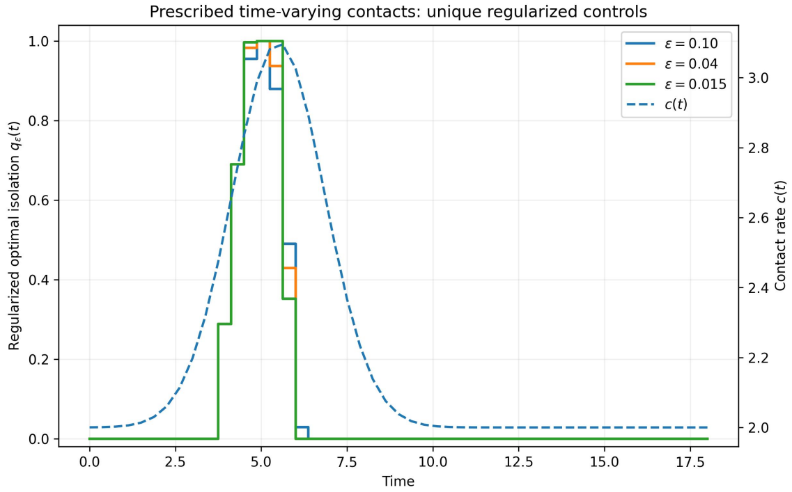
图 9: 给定时变接触率时, 不同 \epsilon 下由原工程离散求解器得到的控制。这里不声称这些离散解全局唯一, 也未证明 \epsilon \downarrow 0 时收敛到原连续问题的最优控制。
