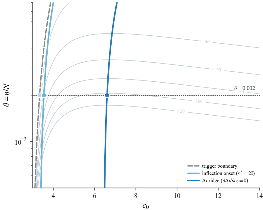
图 24: (\theta, c_0) 平面上阈值控制律的结构相图。三条曲线为触发边界 c_{0,\text{trig}}(\theta) 、内部拐点边界 s^* = 2\bar{s} 与控制时长脊线 \partial \Delta t / \partial c_0 = 0 , 灰色等值线为 \Delta t (天)。图 23 的三个代表 c_0 为三条边界与 \theta = 0.002 (点线) 的交点, 同色圆点标出。本图仅报告结构量, 不含占优边界, 亦不画 J 或 \eta = I_{\text{peak}}^T 参照线。
