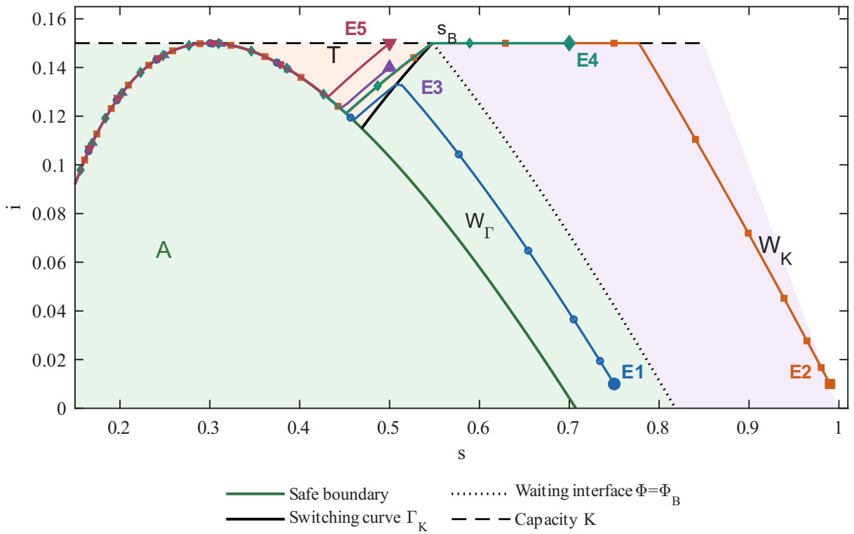
图 1: 不同初值区域及代表轨道的相平面对照。图中标出安全边界、切换曲线 \Gamma_K 、容量线 i = K 、两种等待区的公共边界，以及 E1–E5 的初始状态。理论几何与直接配点轨道采用不同线型或标记。
