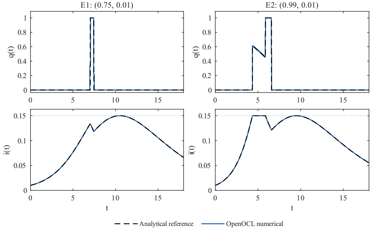
图 2: 两种等待区域下的控制与感染比例：左列为 E1，右列为 E2；上排为 q(t) ，下排为 i(t) 。每幅图比较解析参考与 OpenOCL 结果，数值控制按分段常数形式显示，感染图中的水平线表示容量 K 。
