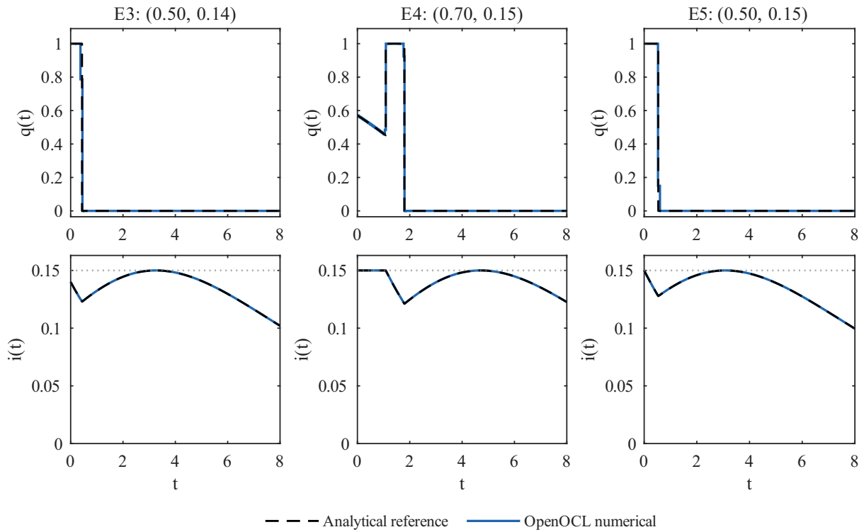
图 3: 立即完全跟踪与容量边界初值的对照。从左到右为 E3、E4、E5，上排为 q(t) ，下排为 i(t) 。解析参考与 OpenOCL 结果的比较重点为初始控制阶段、容量平台是否出现，以及解除位置。
