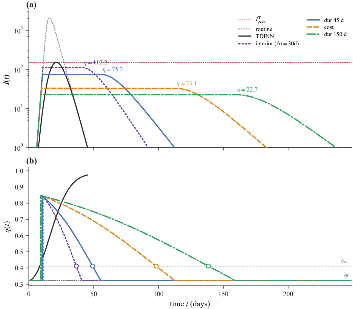
图 21: \eta 杠杆: 固定有效人口 N_{\text{eff}} = 2 \times 10^4 , 沿四条尺度不变边界取阈值 \eta = \theta N_{\text{eff}} 的情景—阈值控制轨迹。各条平台的高度即其 \eta , 已在平台下降转角处直接标出; 四条边界依次为 interior ( \Delta t = 30 \text{ d} , \theta_{\text{int}} = 5.612 \times 10^{-3} , \eta = 112.2 )、dur 45 d ( \theta_{\text{dur45}} = 3.762 \times 10^{-3} , \eta = 75.2 )、cost ( \theta_{\text{cost}} = 1.656 \times 10^{-3} , \eta = 33.1 ) 与 dur 150 d ( \theta_{\text{dur150}} = 1.137 \times 10^{-3} , \eta = 22.7 )。 (a) 社区感染者 I(t) (对数纵轴): 四条平台分别贴合各自的 \eta , 且因 N_{\text{eff}} < N_{45}^* 全部落在 I_{\text{peak}}^T 之下 (红点线)。灰点线为同一 N_{\text{eff}} 下的常规控制; 黑实线为 TDINN 控制, 取西安全市口径下的原始拟合轨迹 (峰值 151.90、清零 45.27 d), 作为固定的现实参照, 不随 N_{\text{eff}} 重算 (见第 8 节 TDINN 基准的口径说明)。 (b) 隔离率 q_c(t) : 四条松弛曲线与 TDINN 的上升高斯 q_{\text{TDINN}}(t) ; 灰点线与灰虚线分别为 q_0 = 0.3230 与拐点高度 q_{\text{inf}} = 1 - 1/[2(1 - \beta)] = 0.4119 。白心圆为各条曲线的凹凸拐点, 均落在 q_{\text{inf}} 上, 与其只依赖 \beta 、不依赖 (N_{\text{eff}}, \eta) 的结论一致。
