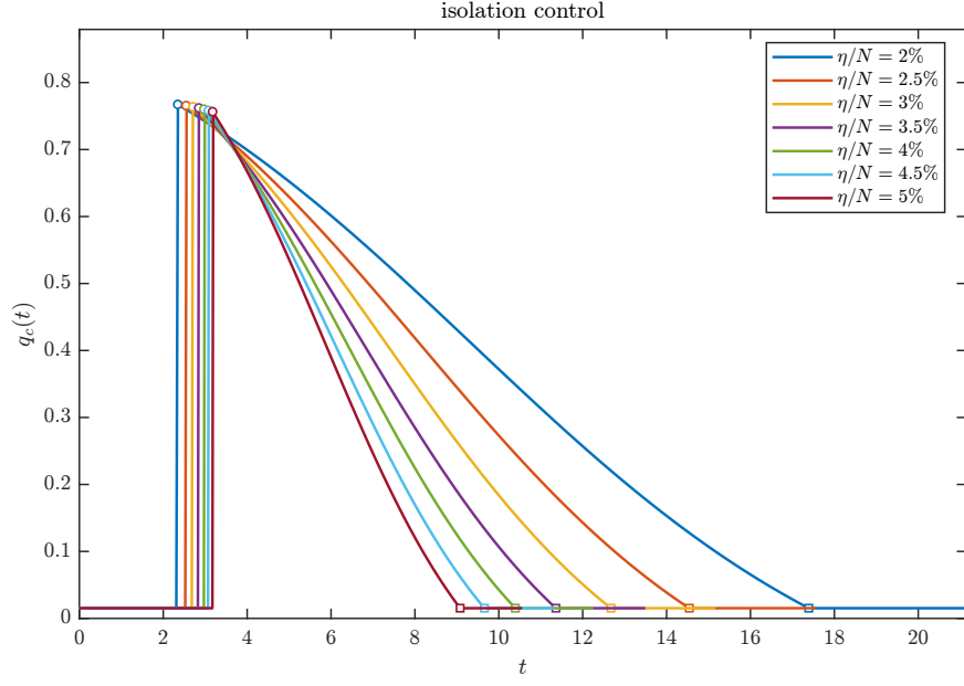
图 6: 情景一中不同 \eta 下隔离率 q_c(t) 的时间轨迹。
