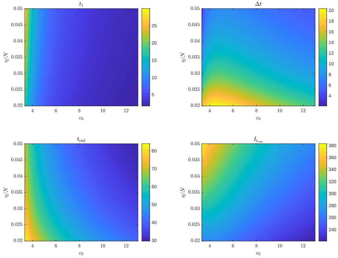
图 9: 情景一中 (c_0, \eta) 平面上的 t_1 、 \Delta t 、 t_{\text{end}} 与 I_{t_{\text{cum}}} 热图。
