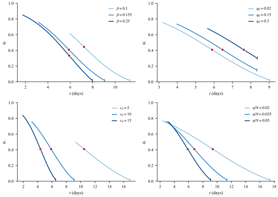
图 2: 四个参数各取低、中、高三值时的隔离控制律 q_c(t) ，横轴为真实时间 t (天)；圆点为拐点，短竖线标出控制解除时刻 t_2 。参数固定同图 1。须注意每条曲线的水平跨度是控制时长 \Delta t ，而曲线整体的左右位置差来自启动时刻 t_1 不同（传播越快 t_1 越早），两者不可混读：例如 c_0 = 15 的曲线靠左且短， c_0 = 5 的靠右且长。
