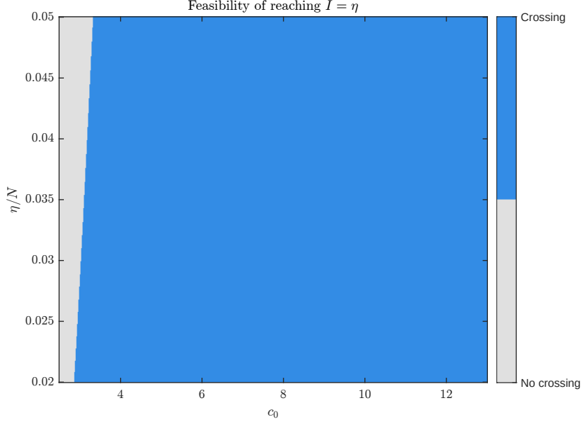
图 10: 情景一中 (c_0, \eta) 平面上是否能够触及 I = \eta 的可行性区域。
