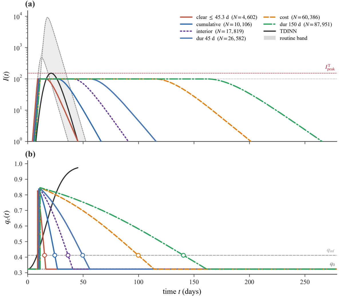
图 22: N 杠杆: 固定绝对阈值 \eta = 100 , 在六个有效人口下的情景一阈值控制轨迹。六条平台高度相同 (均为 \eta ), 故 N_{\text{eff}} 无法在纵轴上直读, 各曲线对应的 N_{\text{eff}} 已随角色名列于图例; 六个取值取自各条边界与 \eta = 100 的交点: clear \leq 45.3 d ( N_{\text{eff}} = 4,602 )、cumulative (10,106)、interior (17,819)、dur 45 d (26,582)、cost (60,386)、dur 150 d (87,951)。(a) I(t) (对数纵轴): 六条平台全部恒在 \eta = 100 (灰虚线), 与池规模无关, 这是强度量只通过 \theta = \eta/N_{\text{eff}} 进入的直接体现; 平台时长则随 N_{\text{eff}} 增大而显著拉长。灰色带为常规控制在 N_{\text{eff}} \in [4,602, 87,951] (与上列六个取值同范围) 上取 8 条几何间隔轨迹的逐点最小-最大包络, 仅绘制到全部成员均未清零为止; 两条灰点线为区间端点的代表轨迹, 因各成员按自身 N_{\text{eff}} 重拟合 I_0 、轨迹相互交叉, 端点轨迹并非处处即为包络。带宽即该反事实策略对池规模的敏感度 (峰值处上下相差约 55 倍), 与阈值控制平台的零带宽形成对照。黑实线为 TDINN 控制的西安全市原始拟合轨迹 (峰值 151.90、清零 45.27 d): 它是已发生的现实控制, 作为固定参照只画一条, 不随 N_{\text{eff}} 重算; 红点线为其峰值 I_{\text{peak}}^T 。(b) q_c(t) : 六条松弛曲线与 TDINN 的 q_{\text{TDINN}}(t) ; 白心圆的拐点同样全部落在 q_{\text{inf}} = 0.4119 , 给出跨 N_{\text{eff}} 的不变性, 与图 21 的跨 \eta 不变性互补。
