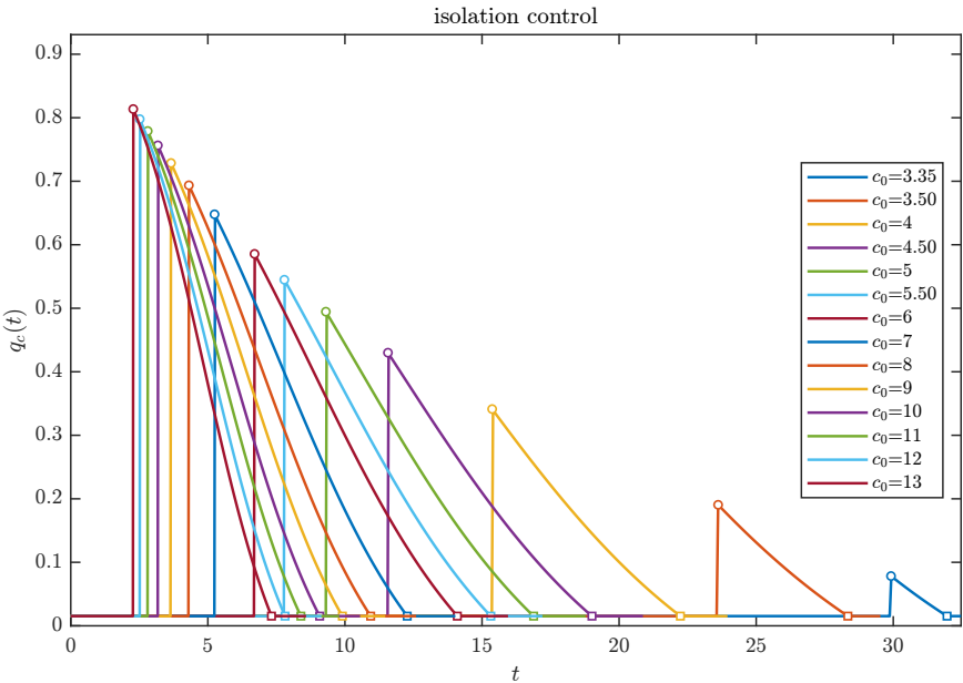
图 5: 情景一中不同 c_0 下隔离率 q_c(t) 的时间轨迹。
