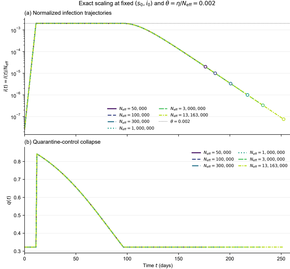
图 17: 固定 (s_0, i_0, \theta = 0.002) 时不同 N_{\text{eff}} 的归一化感染轨迹 i(t) 与隔离率 q(t) 折叠。白心圆为各 N_{\text{eff}} 下绝对判据 I = 1 对应的不同清零终点。
