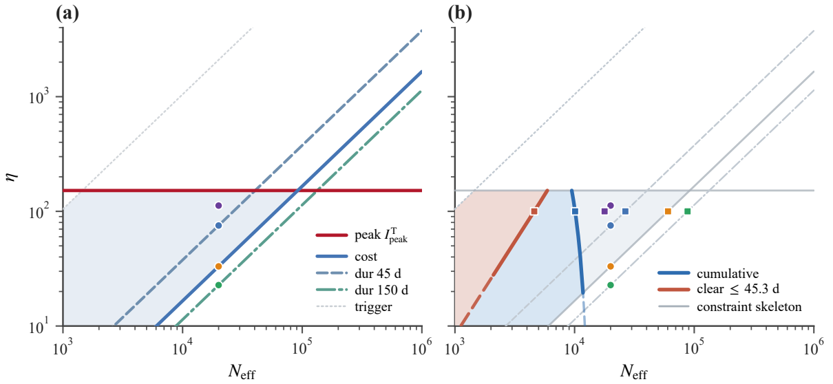
图 20: (N_{\text{eff}}, \eta) 平面上情景一阈值控制相对 TDINN 现实结局的占优区域，双对数坐标。(a) 直线族（强度量）：峰值线 \eta = I_{\text{peak}}^T = 151.90 （红）、成本线 \eta = \theta_{\text{cost}}N （蓝）、两条时长线 \eta = \theta_{\text{dur}}(T_{\text{max}})N （45 d 虚线、150 d 点划线）与触发线 \eta = i_{\text{max}}^{\text{no}}N （点线， i_{\text{max}}^{\text{no}} = 0.1047 ）。阴影为占优楔形 \mathcal{W}_{\text{pcd}} ，以成本线为下界，对应 T_{\text{max}} \rightarrow \infty 口径，顶点 N_{\infty}^* \approx 9.17 \times 10^4 ；由 \theta_{\text{dur}}(T)T \approx 0.170 ， T_{\text{max}} \lesssim 103 d 时改由时长线绑定，例如 N^*(45\text{d}) \approx 4.04 \times 10^4 。(b) 弧线族（广延量）：累计边界（蓝， Nh = I_{\text{rcum}}^T ，自 (9471, 151.90) 到 (12177, 10) ）与清零边界（红， t_{\text{end}} = t_{\text{end}}^T ，自 (2097, 27.89) 到 (5914.3, 151.90) ）；红色内区与蓝色外环互斥填充，故红区即两约束同时满足的区域。累计弧在 (11764, 19.48) 穿出楔形，其后一段以淡虚线示意等值线延续但不再构成 \mathcal{W}_{\text{cum}} 的边界；清零弧在有效池下界 N < I_{\text{rcum}}^T = 2096.76 的一段同样以虚线示意（该区间内广延量比较平凡成立，见第 8.6 节 (4)）。骨架线（峰值·成本·时长·触发）以中性灰重绘以突出弧线。两面板的圆点与方点分别对应图 21 与图 22 的采样角色，同色联动。 \eta = 100 处 N_{\text{cum}} \approx 1.011 \times 10^4 、 N_{\text{clr}} \approx 4.60 \times 10^3 。
