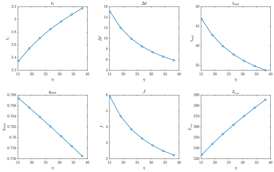
图 8: 情景一中关键指标随 \eta 的变化。
