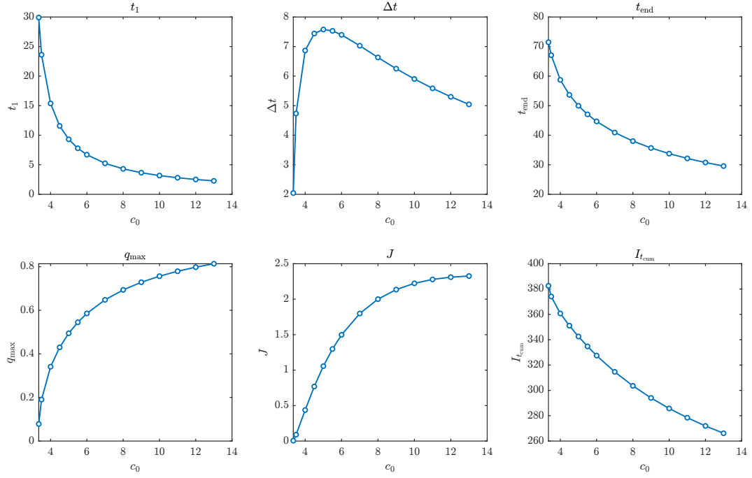
图 7: 情景一中关键指标随 c_0 的变化, 其中扫描范围从 c_{0,\min} + 0.02 延伸至 13。
