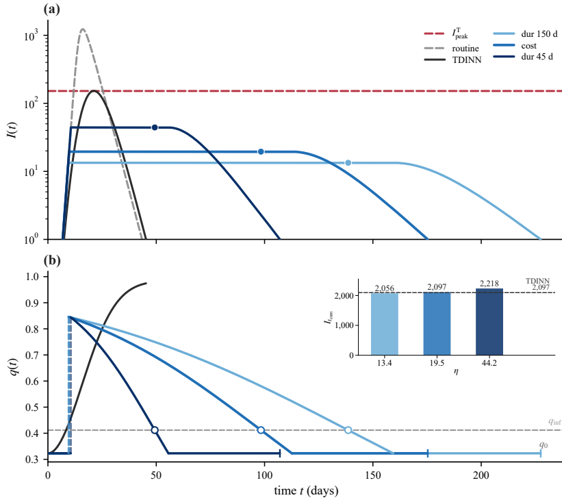
图 25: N_{\text{eff}} = 11,763 \approx N_{\text{cum},\infty}^* 时的 \eta 杠杆。三条参照线的平台高度依次为 \eta = 13.375/19.481/44.246 。右上 inset 给出到动态清零的总累计感染：cost 线恰为 I_{\text{cum}}^T = 2096.76 ——这正是 N_{\text{cum},\infty}^* 的定义（累计弧与成本线的交点）；dur 150 d 低于该参照，dur 45 d 高于该参照。故本图同时给出累计约束的三种情形，而该 N_{\text{eff}} 即累计占优区的上端（第 8.6 小节的窄条 [1.06 \times 10^4, 1.18 \times 10^4] 的右端点）。三条的动态清零时间分别约为 227.5/175.3/107.1 d，仍显著长于 TDINN 的 45.27 d：累计不劣并不蕴含清零不劣。
