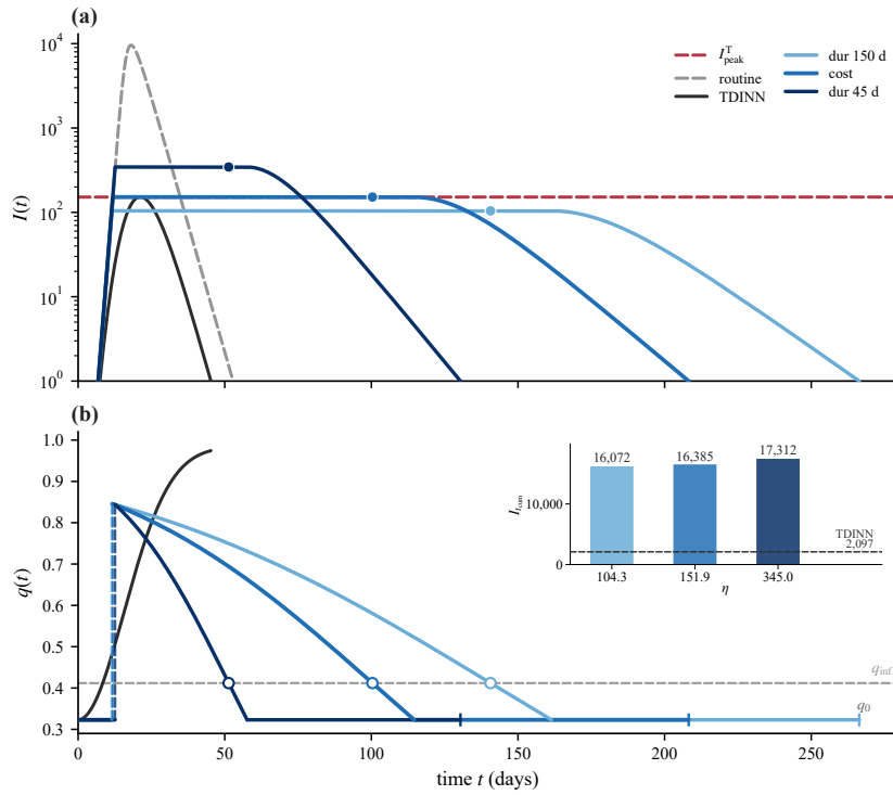
图 27: N_{\text{eff}} = 91,721 \approx N_{\infty}^* 时的 \eta 杠杆。cost 参照线的平台高度 \eta = 151.904 ，恰为 I_{\text{peak}}^T = 151.90 ；dur 45 d 平台 \eta = 345.02 已超过该参照，故峰值约束在该边界上不再成立，而 dur 150 d 平台 ( \eta = 104.295 ) 仍低于参照。
