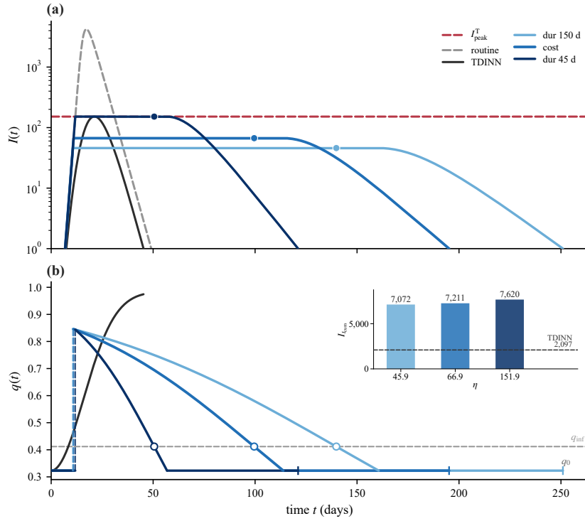
图 26: N_{\text{eff}} = 40,382 \approx N^*(45\text{d}) 时的 \eta 杠杆。dur 45 d 参照线的平台高度 \eta = 151.904 ，恰为 TDINN 峰值参照 I_{\text{peak}}^T = 151.90 ，对应峰值约束的临界情形；dur 150 d 与 cost 平台 ( \eta = 45.918, 66.880 ) 仍位于该参照线下方。
