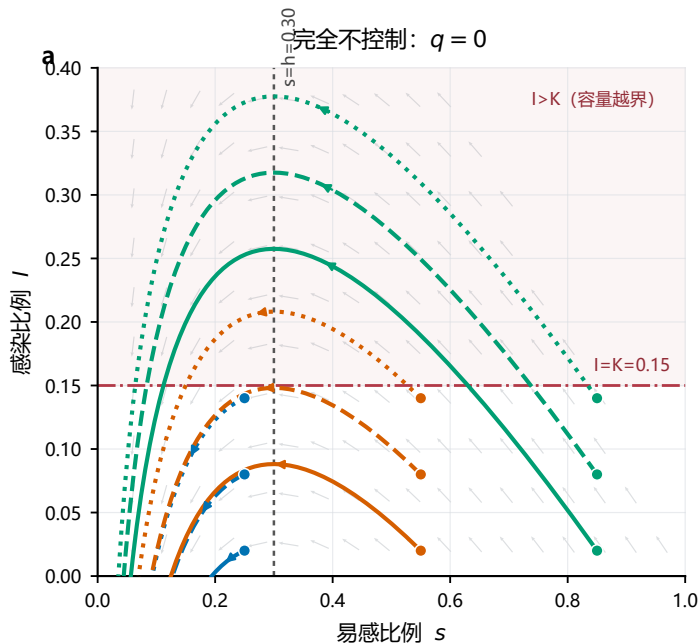
不同初始状态下的极端控制相轨线 基准参数: p=0.5 , c=2 , \gamma=0.3 , K=0.15
