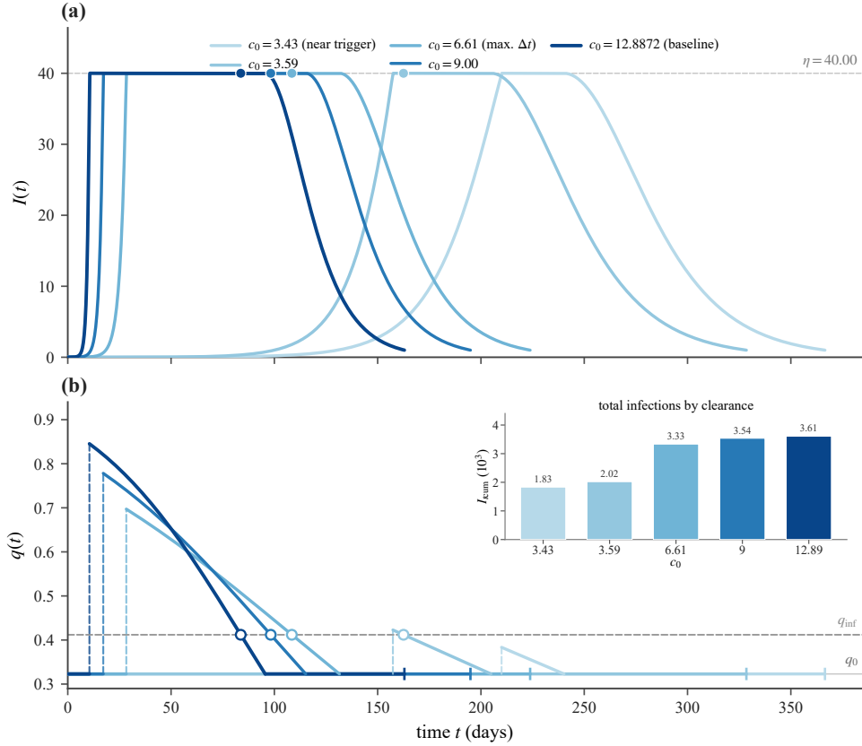
图 24: 固定 N_{\text{eff}} = 2 \times 10^4 、 \theta = 0.002 ( \eta = 40 )、西安传播参数, 沿 c_0 取五个代表值的阈值控制轨迹。(a) I(t) : 平台同高 = \eta , c_0 增大使 t_1 提前、上升支变陡; 实心圆为 q_c(t) 拐点时刻 t_{\text{inf}} 在平台上的投影 ( t_{\text{inf}}, \eta ), 非 I(t) 自身拐点。(b) q_c(t) : q_{\text{max}} 随 c_0 展开, 白圈 (内部拐点) 全部落在 q_{\text{inf}} = 0.4119 ; c_0 = 3.43 因 q_{\text{max}} < q_{\text{inf}} 全程凸、无内部拐点。右上柱图为各情景到自身动态清零 I(t) = 1 的总累计感染 I_{\text{cum}} = I_{c, \text{cum}} + I_{q, \text{cum}} , 在这五个代表点上随 c_0 递增。不画 TDINN 与常规控制: c_0 改变了接触结构, 固定参照不可比。
