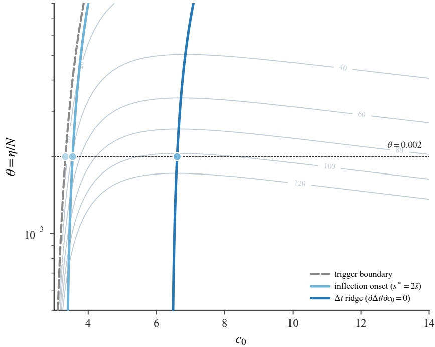
图 25: (\theta, c_0) 平面上阈值控制律的结构相图。三条曲线为触发边界 c_{0,\text{trig}}(\theta) 、内部拐点边界 s^* = 2\bar{s} 与控制时长的极大值线 \partial\Delta t/\partial c_0 = 0 ，灰色等值线为 \Delta t （天）。图 24 的三个代表 c_0 为三条边界与 \theta = 0.002 （点线）的交点，同色圆点标出。本图仅报告结构量，不含占优边界，亦不画 J 或 \eta = I_{\text{peak}}^T 参照线。
