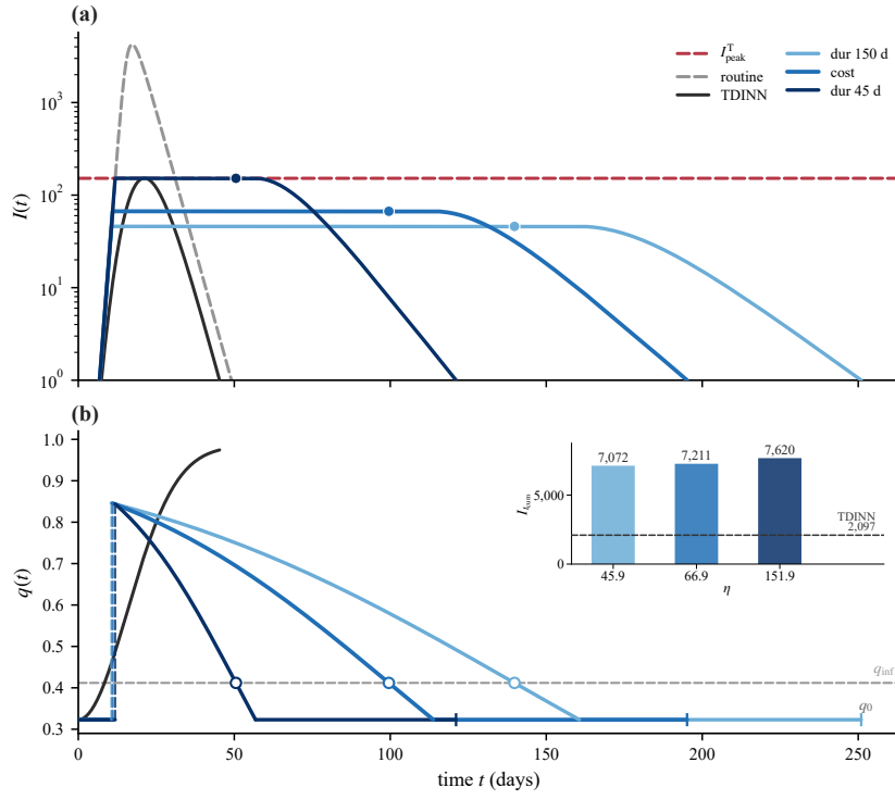
图 27: N_{\text{eff}} = 40,382 \approx N^*(45\text{d}) 时的 \eta 杠杆。dur 45 d 参照线的平台高度 \eta = 151.904 ，恰为 TDINN 峰值参照 I_{\text{peak}}^T = 151.90 ，对应峰值约束的临界情形；dur 150 d 与 cost 平台（ \eta = 45.918 、 66.880 ）仍位于该参照线下方。
