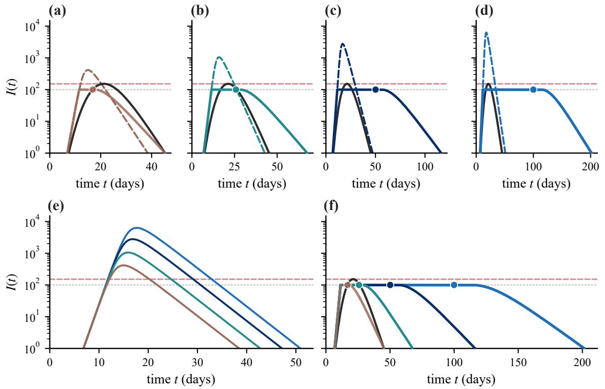
图 23: 图 22 的轨迹分解：仍固定 \eta = 100 ，取其中四个有效人口 \text{clear} \leq 45.3 \text{ d} ( N_{\text{eff}} = 3,970 )、 \text{cumulative} (10,102)、 \text{dur } 45 \text{ d} (26,584)、 \text{cost} (60,381)，把三类 I(t) 按 N_{\text{eff}} 逐条拆开。角色配色、实心圆与两条参照线的含义均同图 22。(a)–(d) 依上列次序各对应一个 N_{\text{eff}} ，每格三条：该 N_{\text{eff}} 的阈值控制（实线）、同一 N_{\text{eff}} 的常规控制（虚线）、固定 TDINN（黑实线）；(e) 只画四条常规控制（均为实线），(f) 只画四条阈值控制与唯一一条 TDINN。六格共用对数纵轴，横轴则各自贴合本格内容，跨格比较时间须读刻度。
