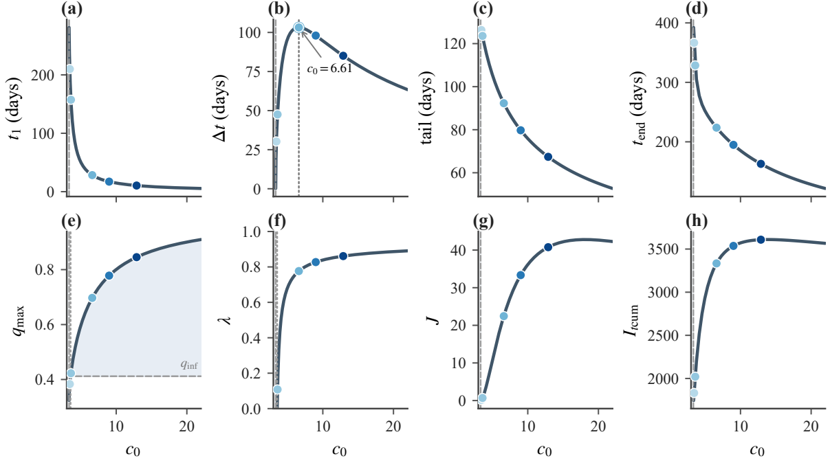
图 29: 固定 N_{\text{eff}} = 2 \times 10^4 、 \theta = 0.002 下阈值控制指标随背景接触率 c_0 的连续扫描。上排为时间分解，三者相加即第四个：(a) 启动时间 t_1 、(b) 平台时长 \Delta t 、(c) 解除控制后的尾段、(d) 清零时刻 t_{\text{end}} = t_1 + \Delta t + \text{尾段} 。下排为结构量与结局量：(e) q_{\text{max}} 、(f) 拐点相对位置 \lambda 、(g) 二次加权成本 J 、(h) 到动态清零的总累计感染 I_{\text{cum}} 。灰色竖线 / 阴影标出触发边界 c_0 = 3.334 、拐点出现边界 c_0 = 3.543 与 \Delta t 脊 c_0 = 6.607 ；同色圆点为图 24 的五个代表 c_0 。四个时间量中只有 \Delta t 非单调，其余三个及 t_{\text{end}} 全程单调递减； J 与 I_{\text{cum}} 各自在 c_0 = 18.1 与 13.9 处取极大后缓降。 J 与 I_{\text{cum}} 仅作该池规模下的结构结果，不叠加任何 TDINN 参照线。
