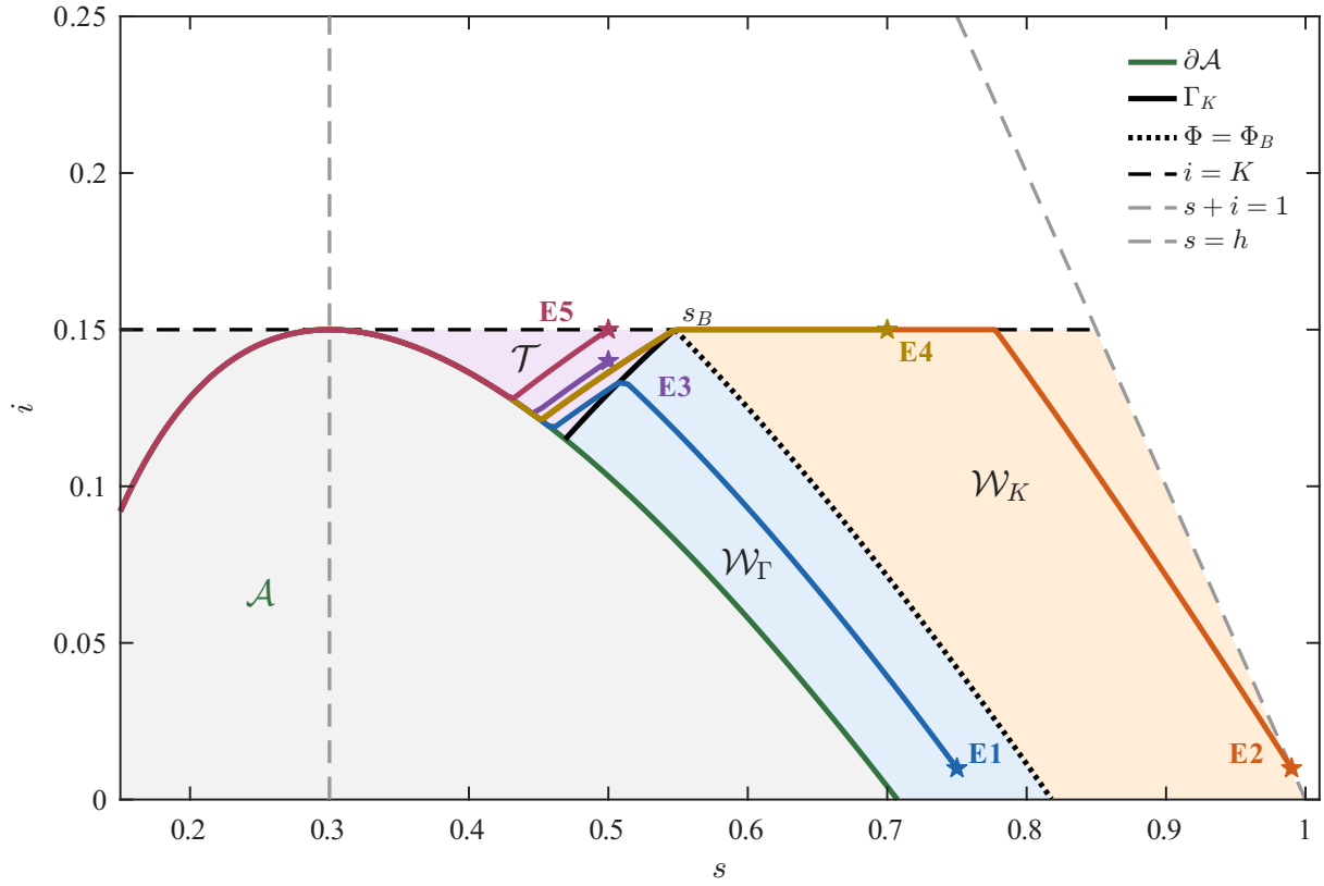
图 1: 不同初值区域及代表轨道的相平面对照。图中标出安全边界、切换曲线 \Gamma_K 、容量线 i = K 、两种等待区的公共边界, 以及 E1–E5 的初始状态。理论几何与直接配点轨道采用不同线型或标记。
