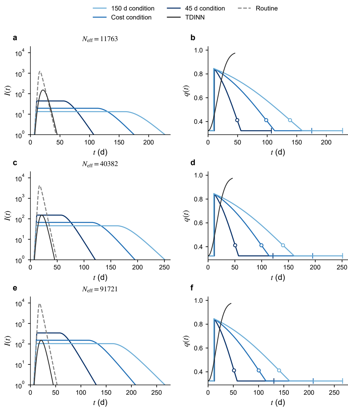
图 18: 三类临界有效人口下的阈值比较。三行依次为 N_{\text{eff}} = 11763, 40382, 91721 ；左列为社区感染者人数（对数纵轴），右列为隔离率。蓝色轨迹对应 150 d 时长、成本和 45 d 时长条件，黑实线为固定 TDINN 参照，灰虚线为同人口常规控制。空心圆标记隔离率拐点，短竖线为清零时刻。
