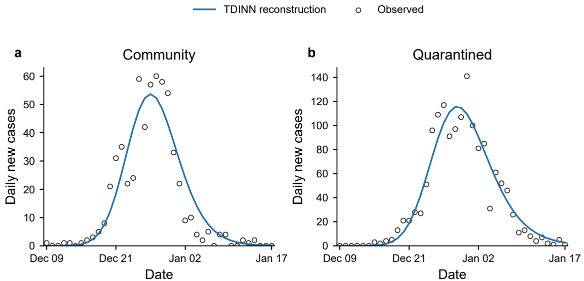
图 9: 西安疫情观测窗口内的日新增病例与 TDINN 重构。(a) 社区发现病例; (b) 隔离发现病例。点为观测值, 实线取自三策略比较所用的同一 TDINN 轨迹, 以相邻整数日累计量之差计算日新增。40 个日区间从 2021 年 12 月 9 日起算; 本图用于拟合重构的比较, 并非独立数据验证。
