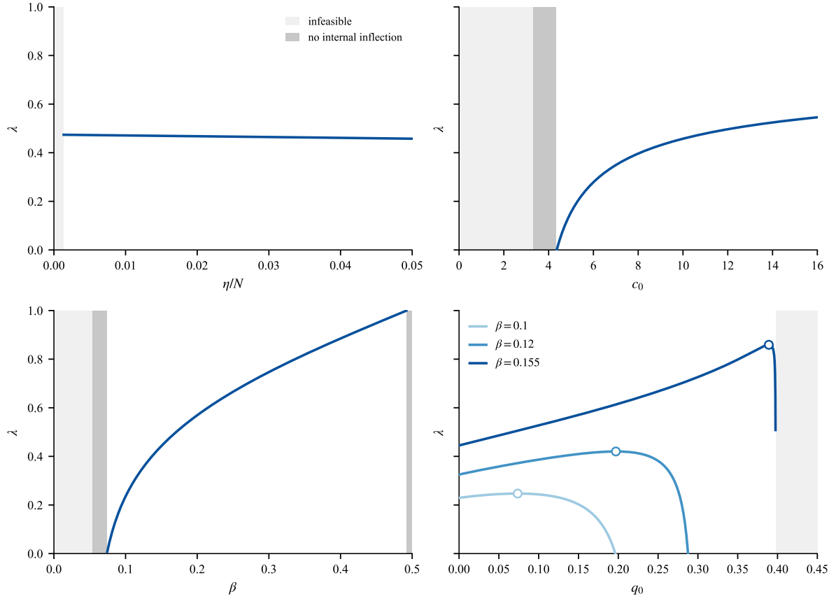
图 4: 拐点相对位置 \lambda 随 \eta/N, c_0, \beta, q_0 的变化。基准取 N = 763, S_0 = 762, I_0 = 1, \beta = 0.155, \gamma = 0.3504, c_0 = 10, q_0 = 0.01526, \eta/N = 0.05 ; q_0 面板另比较 \beta = 0.10, 0.12, 0.155 。空心圆表示数值局部极大值, 浅灰区域表示不满足触发条件, 深灰区域表示已触发控制但无内部拐点。 q_0 面板的灰色区域对应 \beta = 0.155 。
