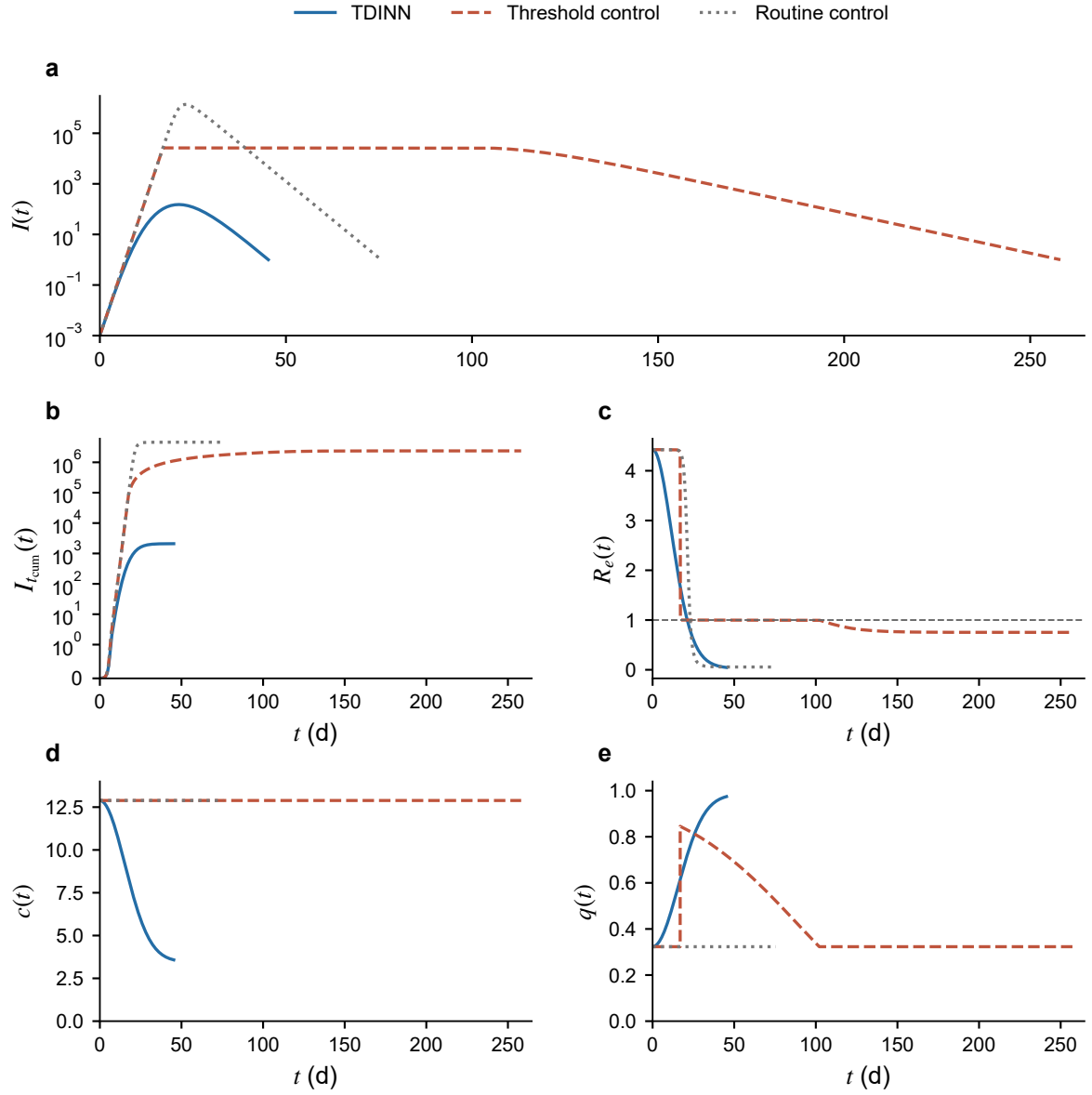
图 10: \eta = 0.002N 时三策略的全过程比较。(a) 社区感染者人数 I(t) ; (b) 总累计感染 I_{cum}(t) ; (c) 有效再生数 R_e(t) ; (d) 接触率 c(t) ; (e) 隔离率 q(t) 。各轨迹分别画至自身的动态清零时刻, 横轴使用同一时间原点。(a) 为对数纵轴, (b) 为保留零值的对称对数纵轴 (线性区阈值为 1 人); (c) 的水平虚线为 R_e = 1 。
