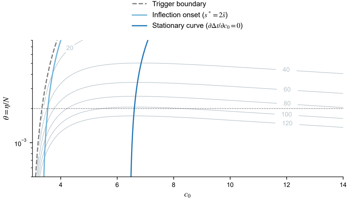
图 16: (\theta, c_0) 平面上的触发边界、内部拐点边界 s^* = 2\bar{s} 和控制持续时间驻点曲线 \partial\Delta t/\partial c_0 = 0 。灰色等值线表示控制持续时间，水平点线为 \theta = 0.002 。
