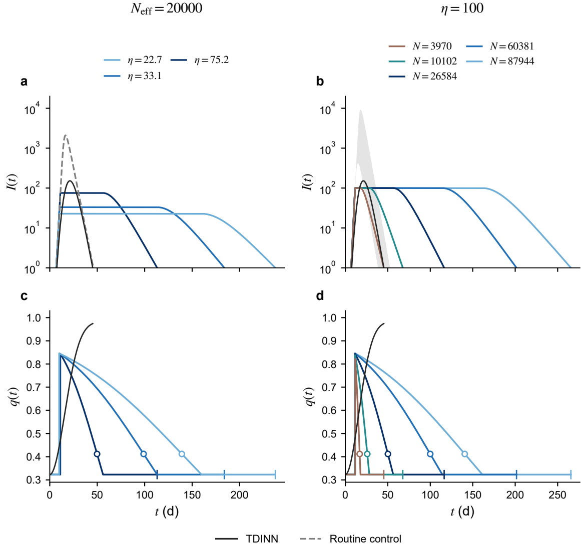
图 14: 阈值与有效人口对轨迹的不同影响。左列固定 N_{\text{eff}} = 20000 ， \eta = 22.7, 33.1, 75.2 分别对应 150 d 时长、成本和 45 d 时长条件；右列固定 \eta = 100 ，保留全部五个人口规模，其中 3970, 10102 低于 N_{\text{floor}} ，仅用于展示边界外的轨迹。(a)、(b) 为社区感染者人数；(c)、(d) 为隔离率。黑实线为固定 TDINN 参照；左列灰虚线为同人口常规控制，右列灰带为常规轨迹范围。空心圆只标在隔离率曲线的拐点处，短竖线表示动态清零时刻。
