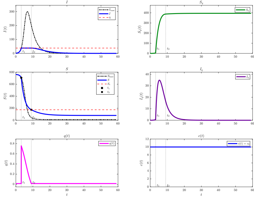
图2: 仅隔离阈值控制与常规控制的时间轨迹。参数为 N = 763 、 S_0 = 762 、 I_0 = 1 、 S_q(0) = I_q(0) = R(0) = 0 、 \beta = 0.155 、 c_0 = 10 \text{ d}^{-1} 、 q_0 = 0.01526 、 \gamma = \delta_q = 0.3504 \text{ d}^{-1} 、 \eta = 0.05N = 38.15 。此处的阈值比例用于说明解析结果，不作具体 ICU 容量换算。阈值控制在 [t_1, t_2] 内维持 I = \eta ， q_c 从启动最大值下降至 q_0 ； c(t) 始终为 c_0 。横轴为自初始时刻起的天数。
