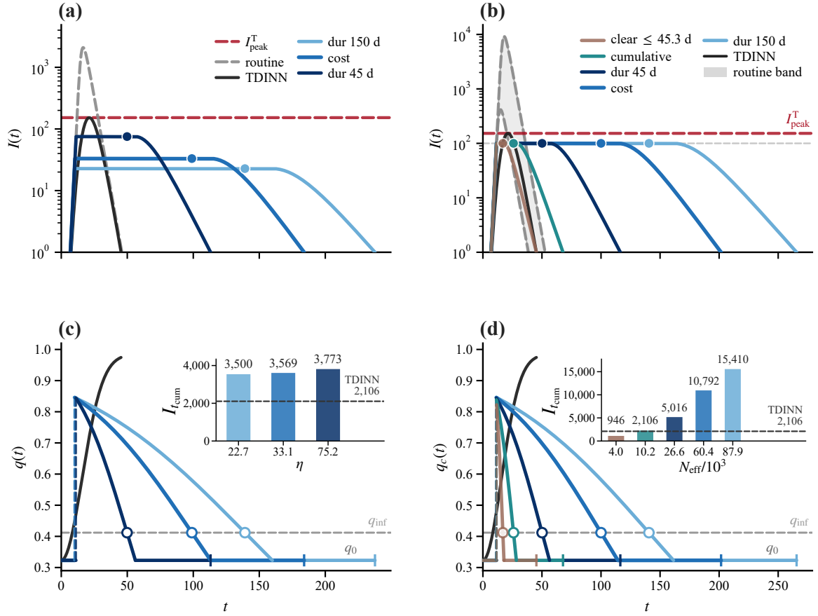
图 18: 阈值与有效人口对轨迹的不同影响。左列固定 N_{eff} = 20000 , \eta = 22.7, 33.1, 75.2 分别对应 150 d 时长、成本和 45 d 时长条件；右列固定 \eta = 100 , 清零、累计感染、45 d 时长、成本和 150 d 时长条件分别对应 N_{eff} \approx 3973, 10151, 26584, 60424, 87944 。前两个人口规模低于 N_{floor} , 仅用于展示边界外的轨迹。(a)、(b) 为社区感染者人数；(c)、(d) 为隔离率；横轴 t 的单位为天。黑实线为固定 TDINN 参照，红虚线为其感染峰值；左列灰虚线为同人口常规控制，右列灰带为常规轨迹范围。空心圆标记隔离率拐点，水平段上的实心点是该时刻在感染曲线上的投影，并非感染曲线自身的拐点；短竖线表示动态清零时刻。内嵌柱图给出清零时的总累计感染，虚线为 TDINN 参照 2105.63。
