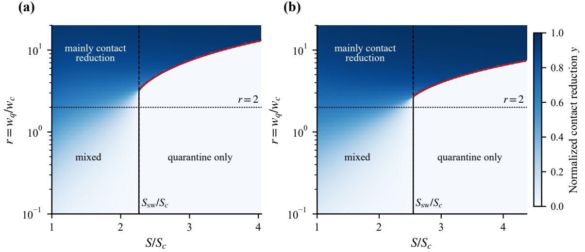
图 11: 固定 w_c = 1 、改变 r = w_q/w_c 时的类内最低二次成本分配。(a) 基准参数；(b) 西安参数。颜色为 y = (1 - c_c^*/c_0)/(1 - S_c/S) ； y = 0 为仅隔离端点， y = 1 为仅减少接触端点。竖直虚线为端点局部判据 S_{sw}/S_c ，黑色区域边界及红色线为数值候选比较所支持的全局选择边界，二者不能混同；水平点线为默认 r = 2 。横轴从左向右为 S 增大方向，与控制时间的先后相反；退出端点不作为份额验证数据。
