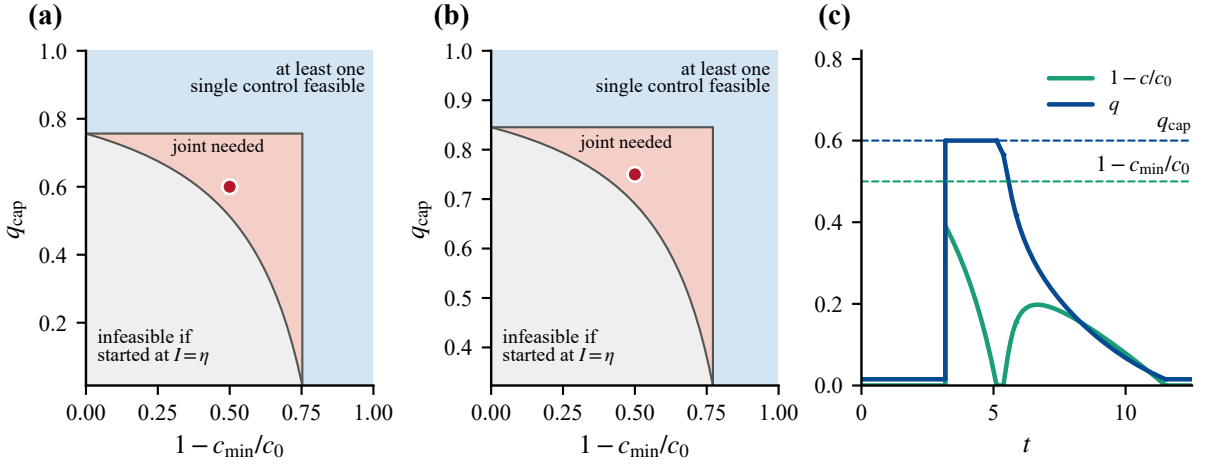
图 10: 能力限制下的可行区域与代表轨迹。(a) 基准参数；(b) 西安参数。横轴为最大接触减少比例 1 - c_{\text{min}}/c_0 ，纵轴为隔离比例上限 q_{\text{cap}} ；灰色、浅红色、浅蓝色分别表示规定触发状态下不可行、两种单控制均不可行但联合可行、至少一种单控制可行。边界等号归入可行侧， q_{\text{cap}} = 1 只作为坐标框上缘，不作为额外能力上限的样例。红点为与计算轨迹共用配置的代表能力组合。(c) 基准代表点的受限最低二次成本分配，绘至名义退出后 1 天；完整清零轨迹保留在计算输出中，横轴 t 的单位为天。
