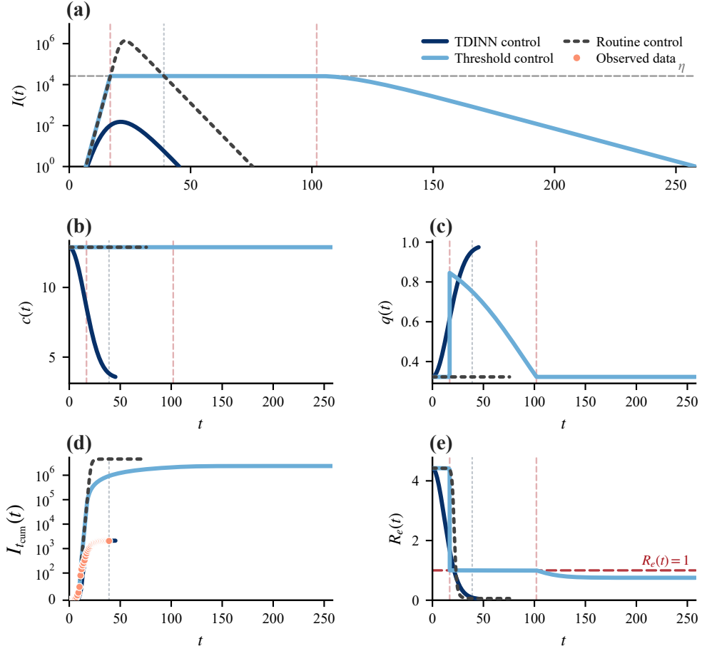
图 10: \eta = 0.002N 时三策略的全过程比较。(a) 社区感染者人数 I(t) ; (b) 接触率 c(t) ; (c) 隔离率 q(t) ; (d) 总累计感染 I_{\text{cum}}(t) ; (e) 有效再生数 R_e(t) 。各轨迹分别画至自身的动态清零时刻, 横轴使用同一时间原点, t 的单位为天。(a) 为对数纵轴; (d) 为对称对数纵轴 (线性区阈值为 100 人), 散点为观测累计量; (e) 的水平虚线为 R_e = 1 。浅红色竖虚线标记控制启动与解除, 灰色竖点线标记观测窗口结束。
