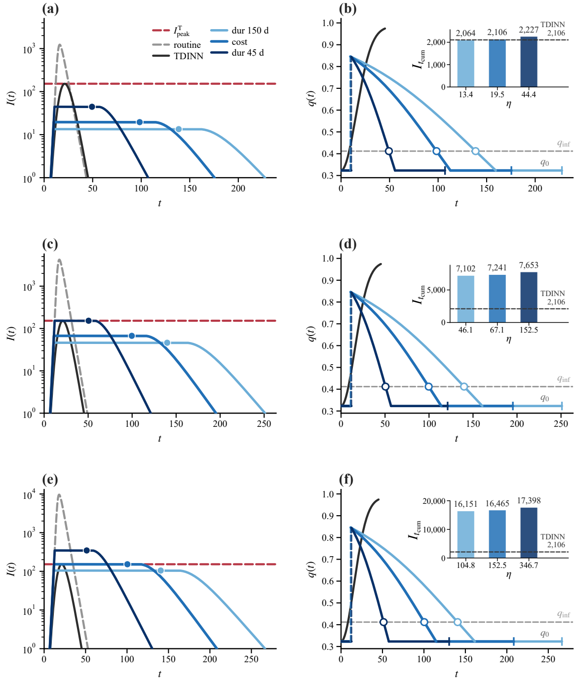
图 22: 三类临界有效人口下的阈值比较。三行依次为 N_{\text{eff}} = 11813, 40553, 92174 ; 左列为社区感染者人数 (对数纵轴), 右列为隔离率, 横轴 t 的单位为天。(a) 中的图例适用于三行: 蓝色轨迹对应 150 d 时长、成本和 45 d 时长条件, 黑实线为固定 TDINN 参照, 灰虚线为同人口常规控制, 红虚线为 TDINN 感染峰值。空心圆标记隔离率拐点, 水平段上的实心点为该时刻在感染曲线上的投影而非感染曲线的拐点, 短竖线为清零时刻。内嵌柱图给出清零时的总累计感染, 虚线为 TDINN 参照 2105.63。
