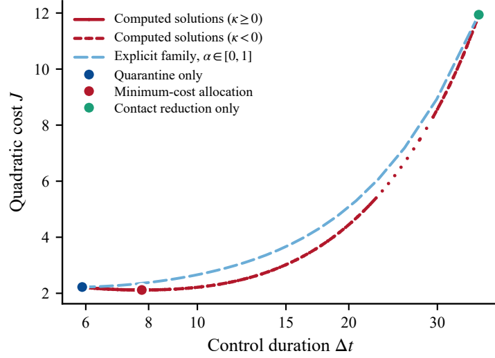
图 12: 基准参数下二次成本与控制持续时间的关系。红色曲线连接已核查的 J + \kappa\Delta t 最小化解，实线与短虚线分别对应 \kappa \geq 0 和 \kappa < 0 ；相邻计算点时长间距较大处不连线；连线不表示中间时长已有匹配乘子。浅蓝虚线为显式 \alpha 族，圆点为两种单控制与无时长限制的最低成本分配。横轴为对数坐标， \Delta t 与 J 的单位均为天。
