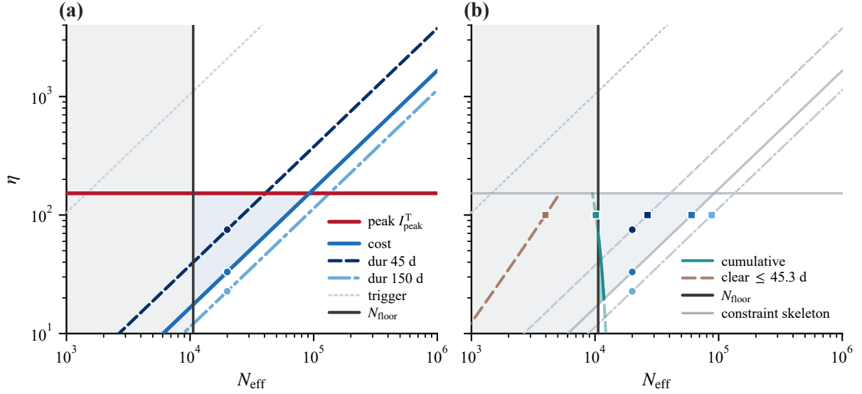
图 17: 西安参数下 (N_{\text{eff}}, \eta) 平面比较区域的近似展示。(a) 峰值条件及成本、时长和触发参考直线；后三者采用 N_{\text{ref}} = 13,163,000 下的未取整比例。人口下界右侧的浅蓝区域示意峰值、成本与触发条件的交集，未另加时长上限；左侧灰色区域因 N < N_{\text{floor}} 被排除。(b) 加入累计感染和清零时间的等值曲线。竖直实线为 N_{\text{floor}} = 1.06 \times 10^4 。计算所得累计感染与成本条件的交点约为 (11813, 19.55) ，清零时间等值曲线位于人口下界左侧。圆点和方点分别示意固定人口改变阈值、固定阈值改变人口的两类比较；轨迹案例的具体参数见图 18(a,c)、18(b,d)。
